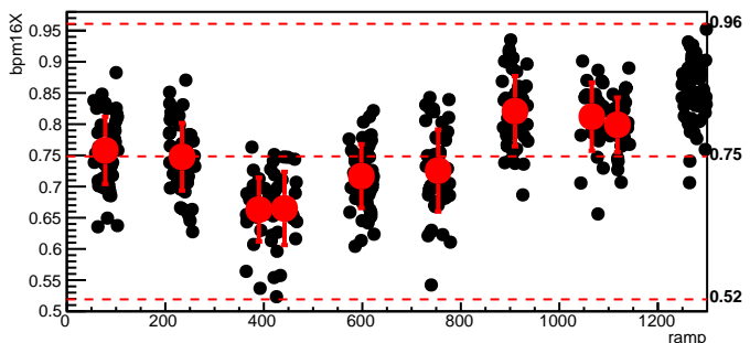
bmod_trim5,cyc=10369
