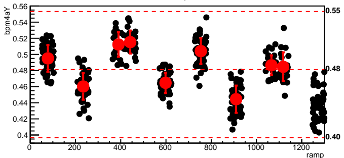
bmod_trim3,cyc=10369
