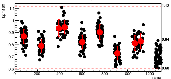
bmod_trim3,cyc=10369
