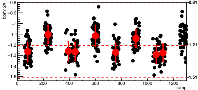
bmod_trim6,cyc=10369
