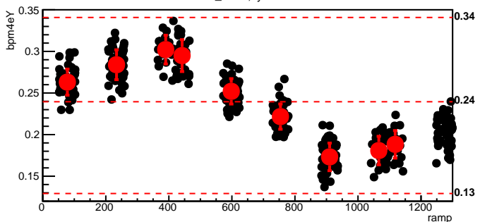
bmod_trim2,cyc=10369
