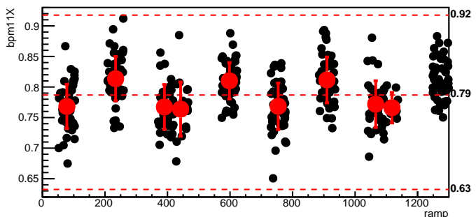
bmod_trim4,cyc=10369
