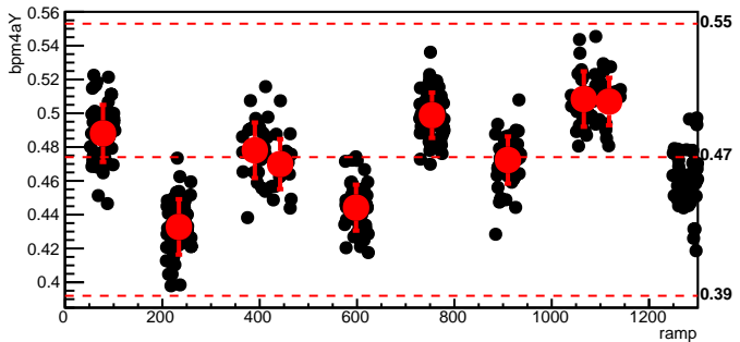
bmod_trim7,cyc=10369
