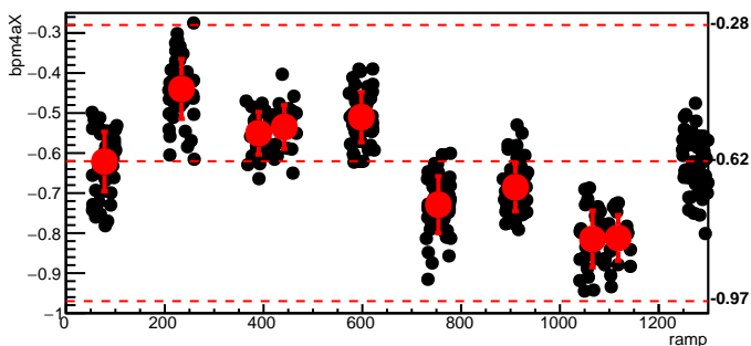
bmod_trim7,cyc=10369
