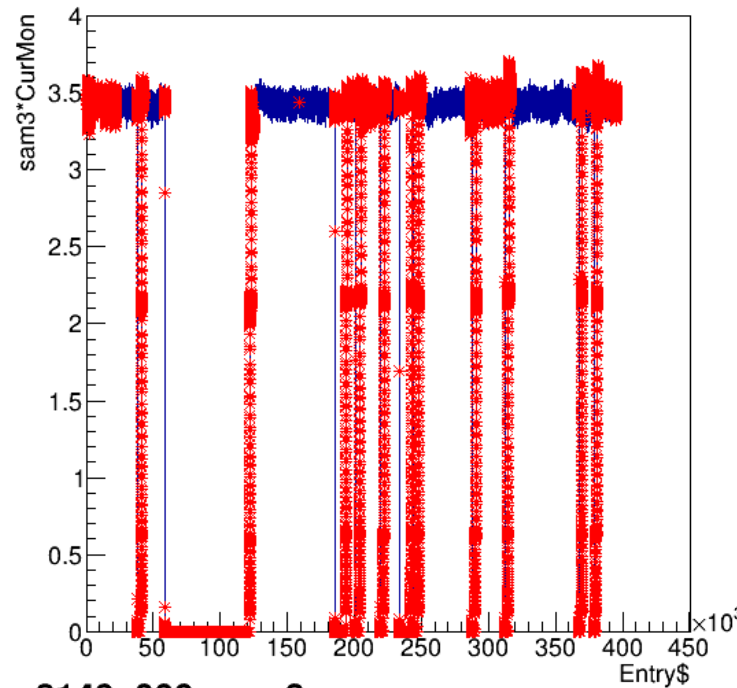
sam3*CurMon:Entry$
