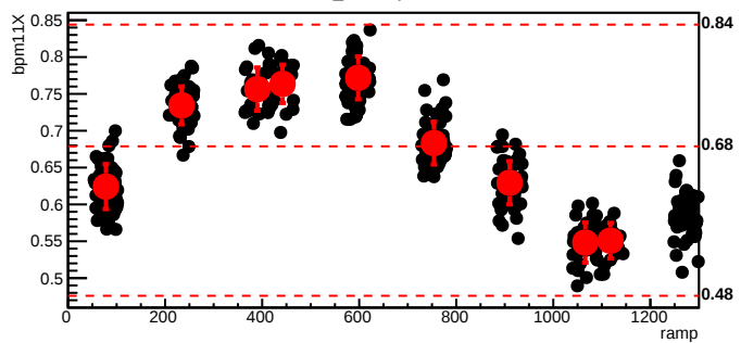
bmod_trim5,cyc=10516
