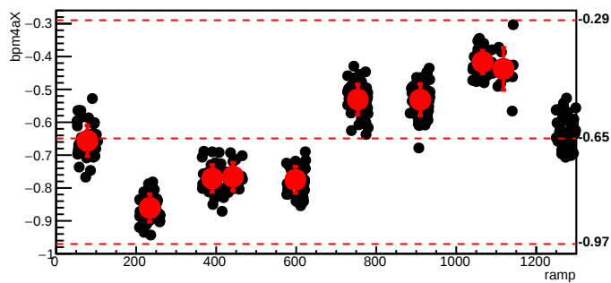
bmod_trim1,cyc=10516
