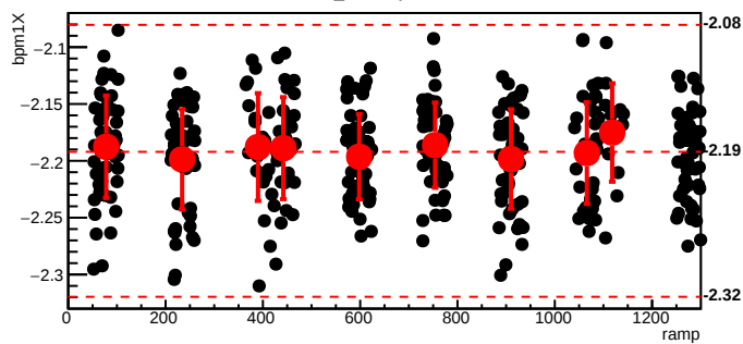
bmod_trim2,cyc=10523
