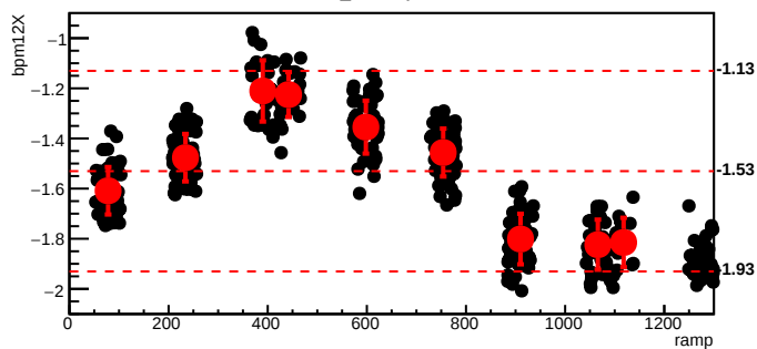
bmod_trim5,cyc=10523
