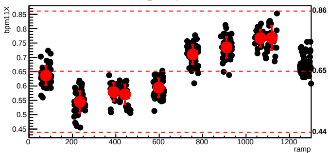
bmod_trim7,cyc=10523
