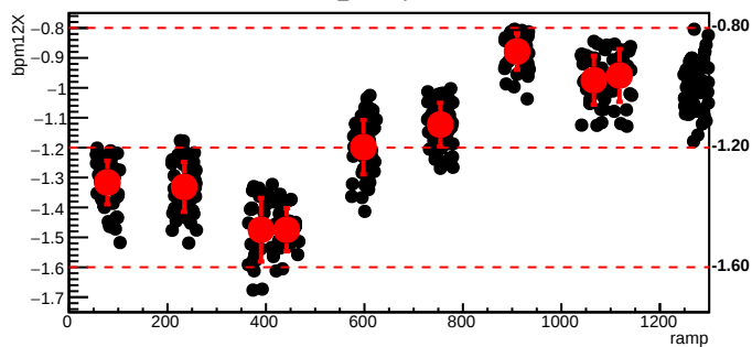
bmod_trim7,cyc=10524
