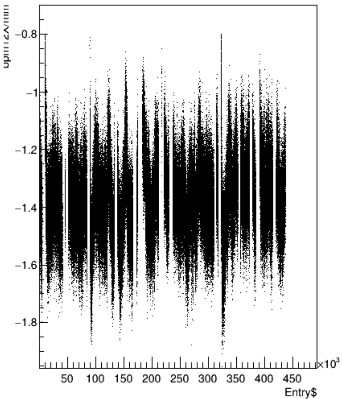
bpm12X/mm:Entry$ {ErrorFlag==0}
