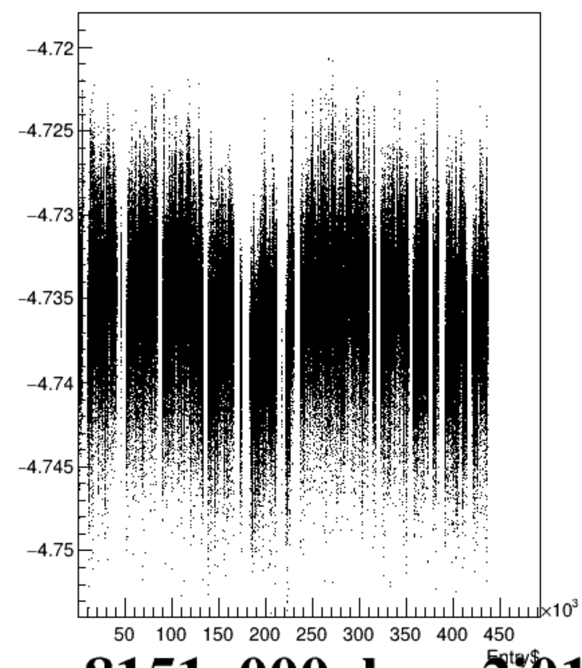
bpm2i01Y/mm:Entry$ {ErrorFlag==0}
