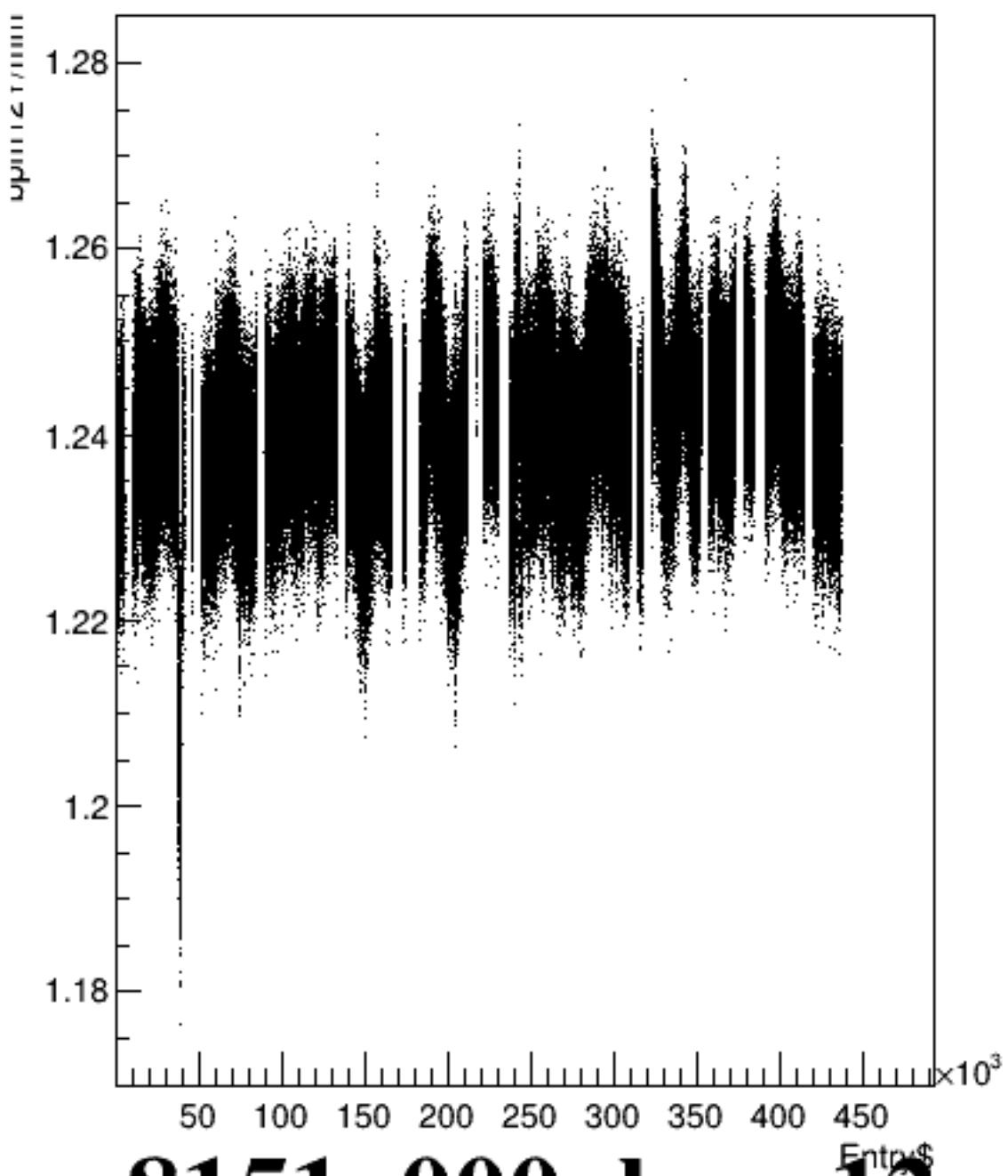
bpm12Y/mm:Entry$ {ErrorFlag==0}
