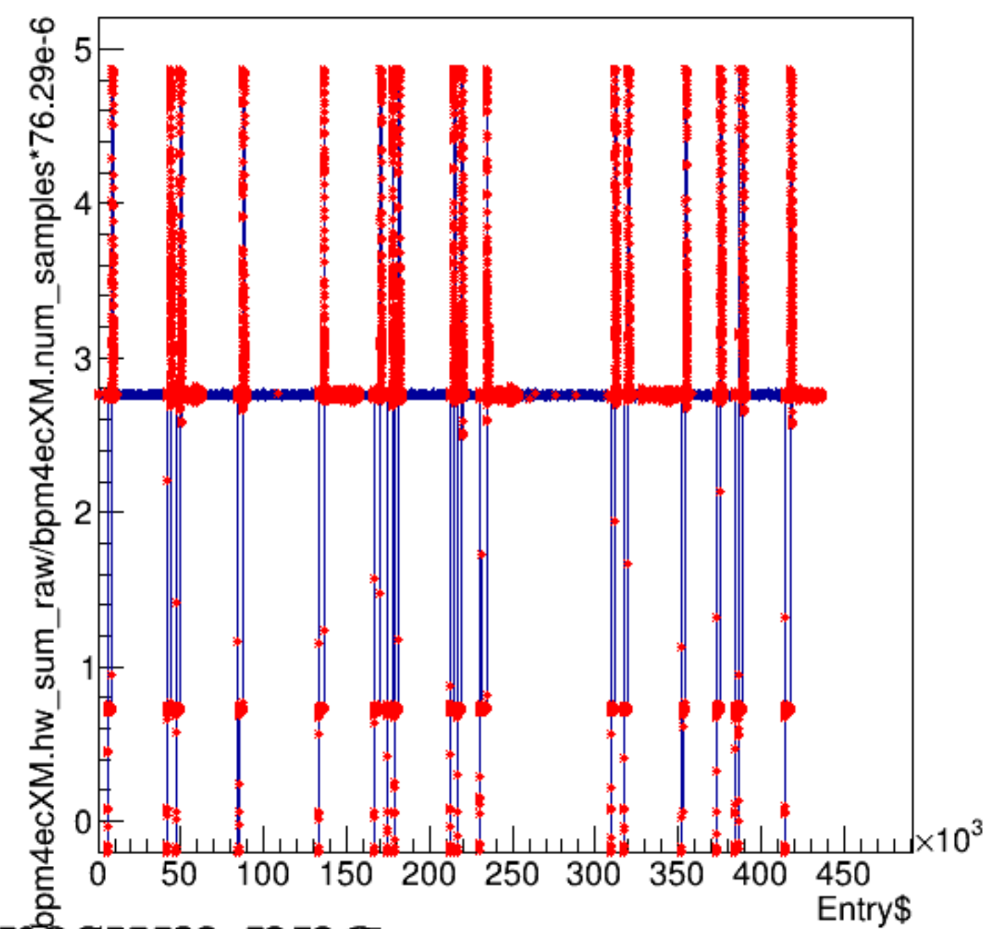
bpm4ecXM.hw_sum_raw/bpm4ecXM.num_samples*76.29e-6:Entry$
