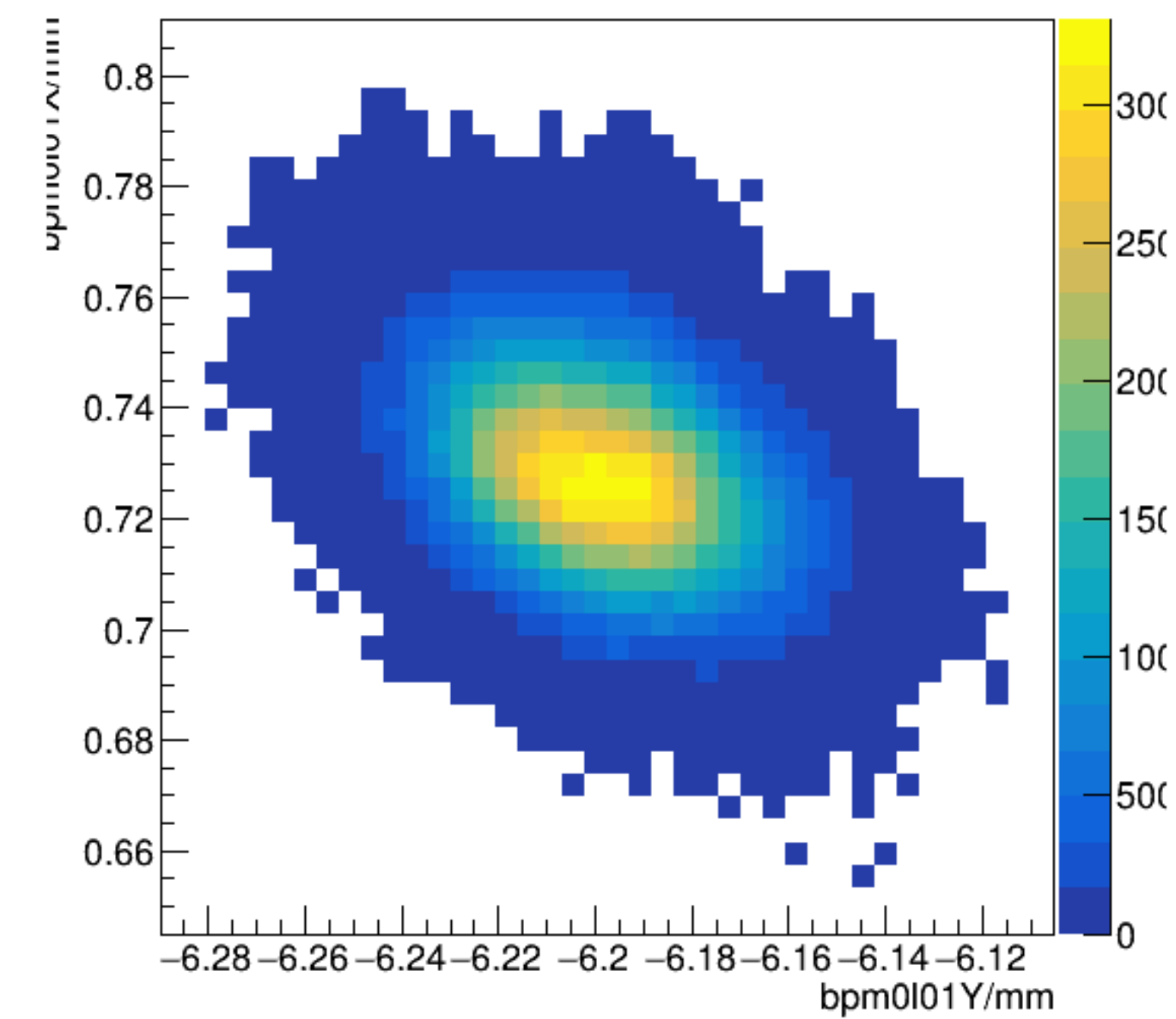
bpm0l01X/mm:bpm0l01Y/mm {ErrorFlag==0}
