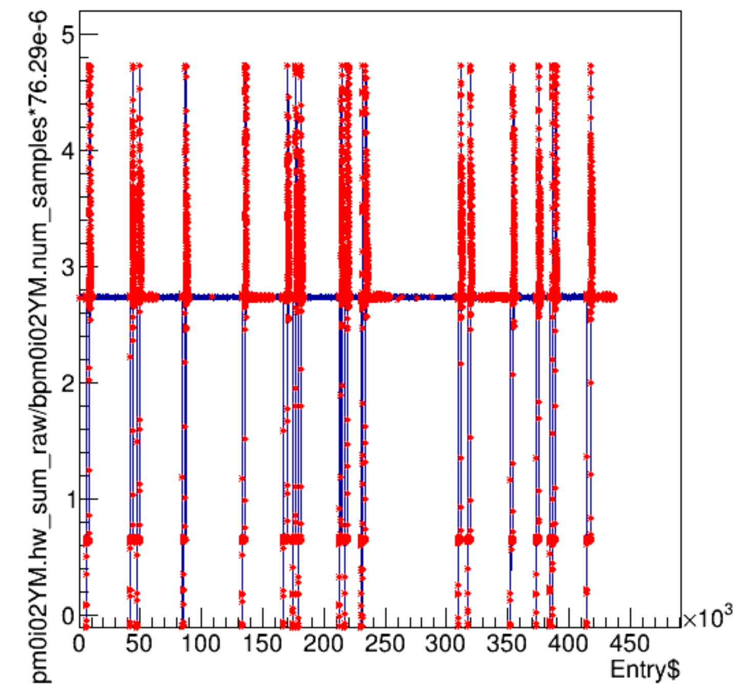
bpm0i02YM.hw_sum_raw/bpm0i02YM.num_samples*76.29e-6:Entry$
