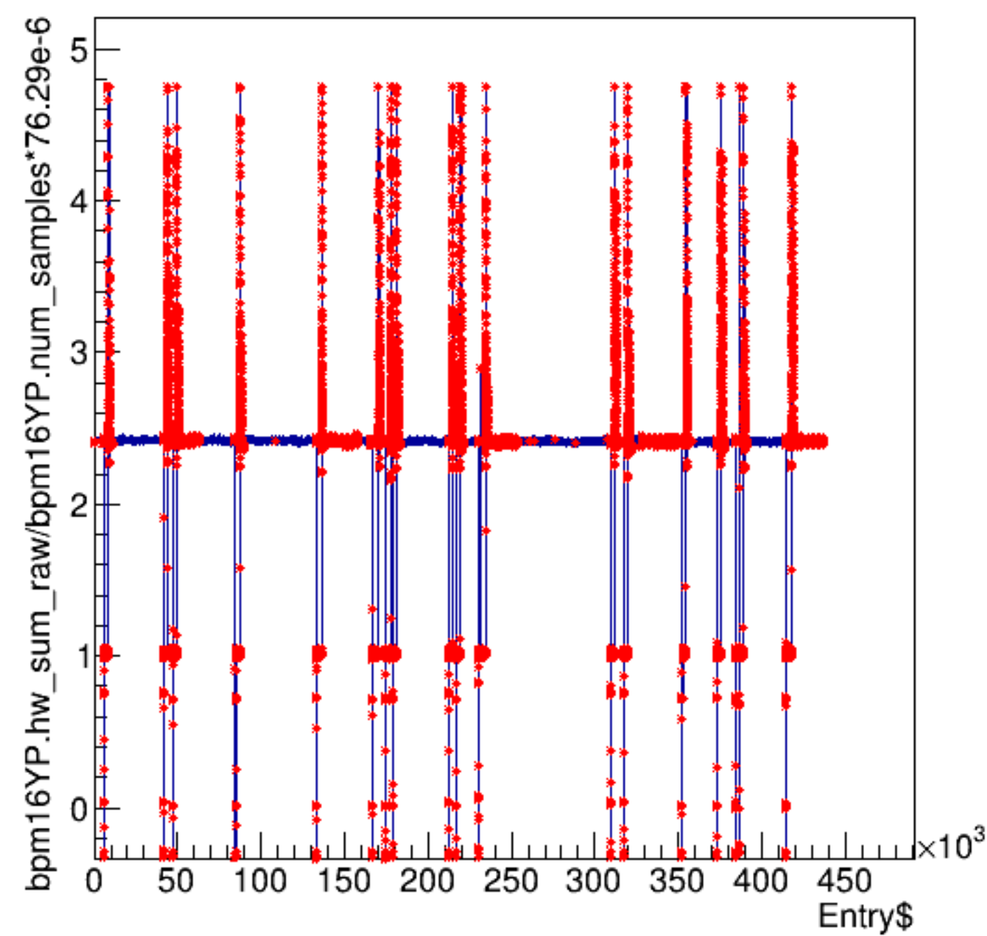
bpm16YP.hw_sum_raw/bpm16YP.num_samples*76.29e-6:Entry$
