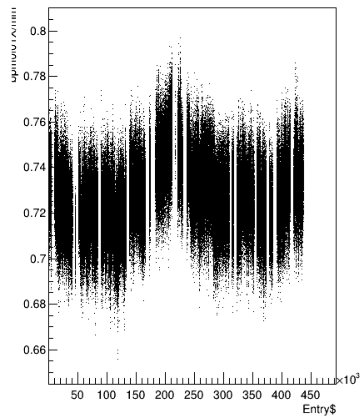
bpm0l01X/mm:Entry$ {ErrorFlag==0}
