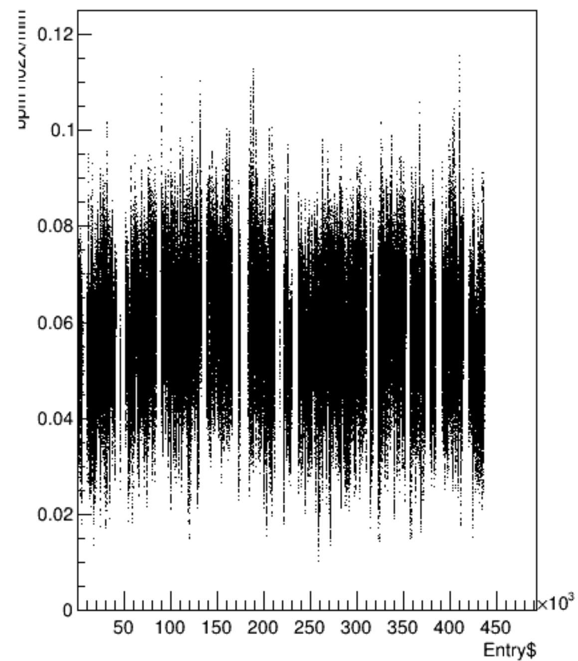
bpm1i02X/mm:Entry$ {ErrorFlag==0}
