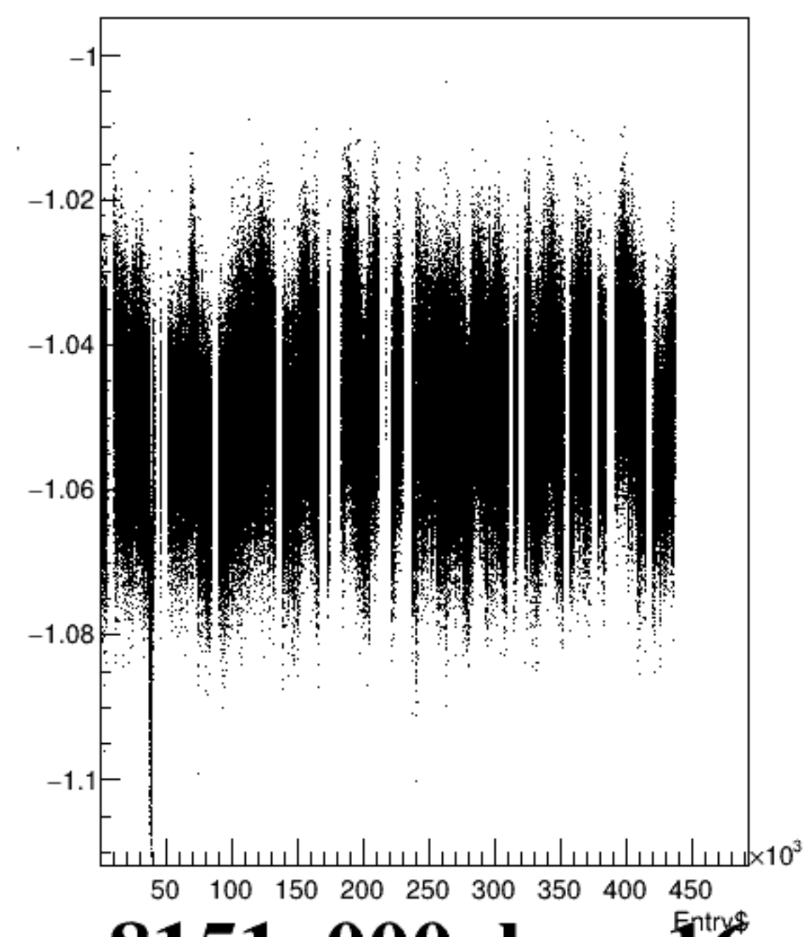
bpm16Y/mm:Entry$ {ErrorFlag==0}
