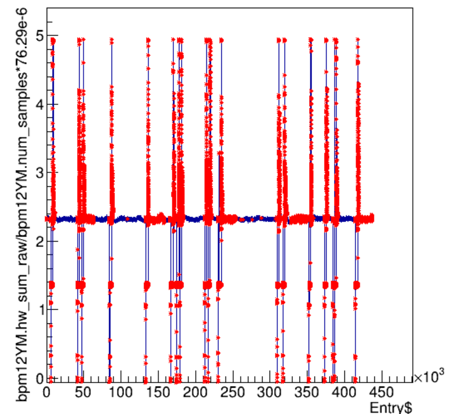
bpm12YM.hw_sum_raw/bpm12YM.num_samples*76.29e-6:Entry$
