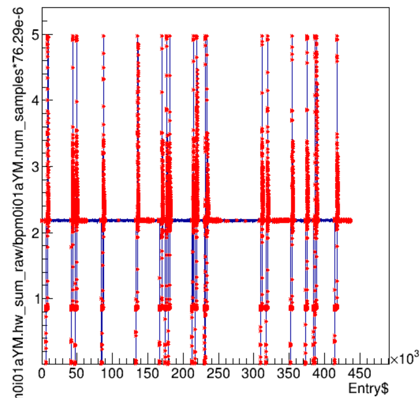
bpm0i01aYM.hw_sum_raw/bpm0i01aYM.num_samples*76.29e-6:Entry$
