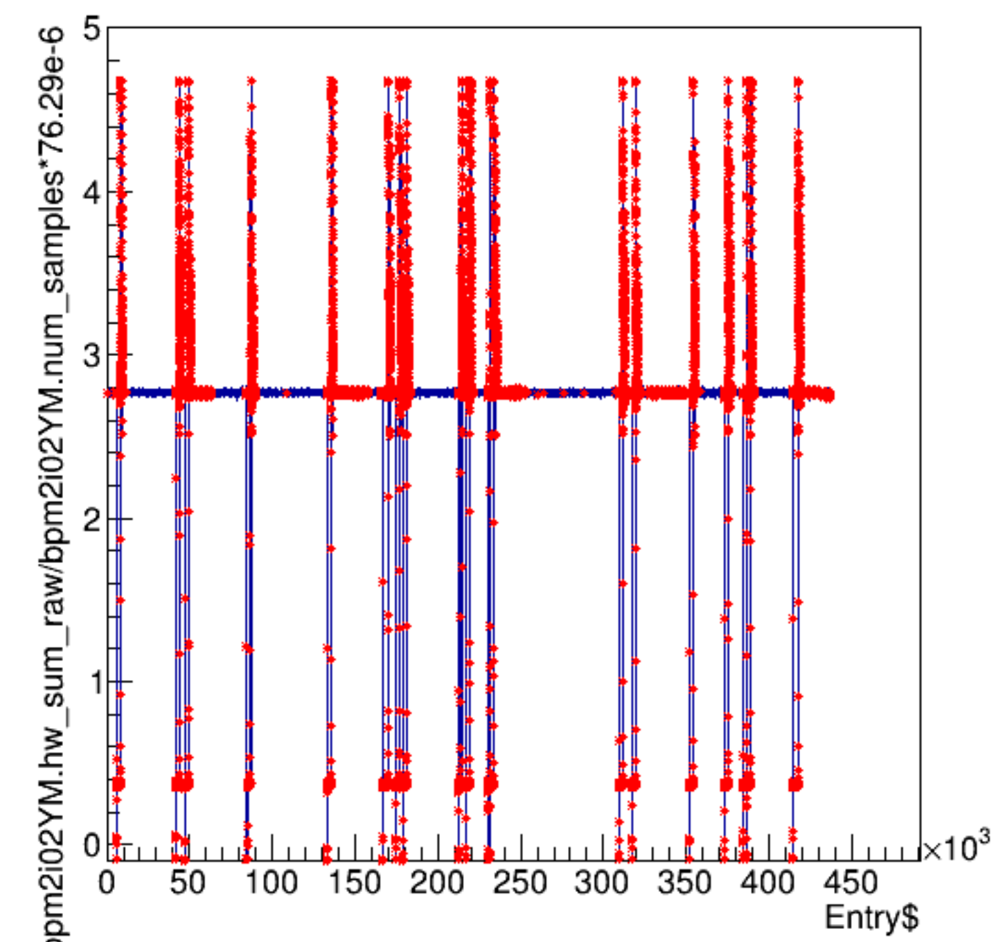
bpm2i02YM.hw_sum_raw/bpm2i02YM.num_samples*76.29e-6:Entry$
