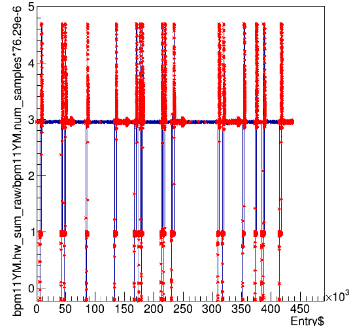
bpm11YM.hw_sum_raw/bpm11YM.num_samples*76.29e-6:Entry$
