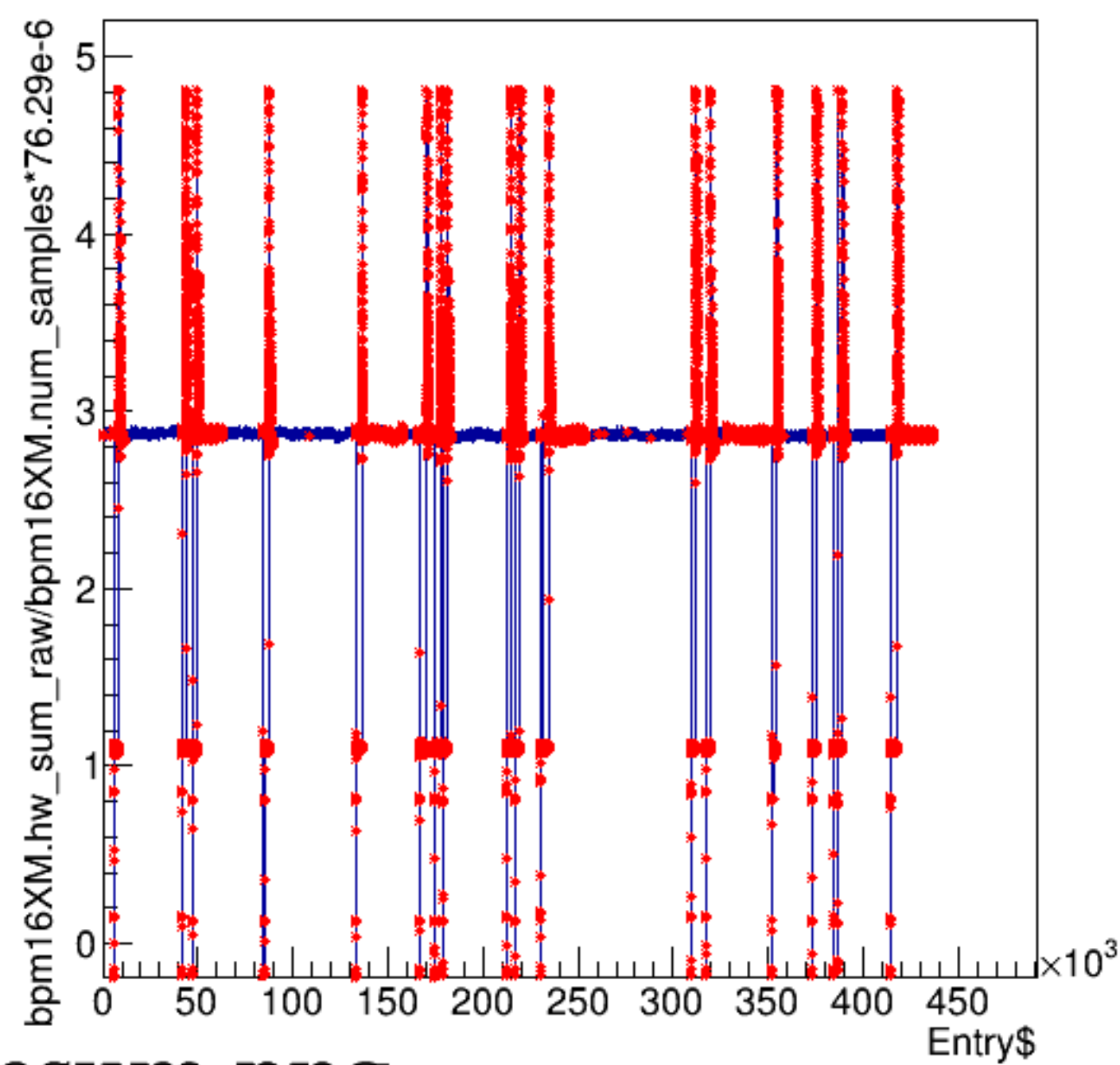
bpm16XM.hw_sum_raw/bpm16XM.num_samples*76.29e-6:Entry$
