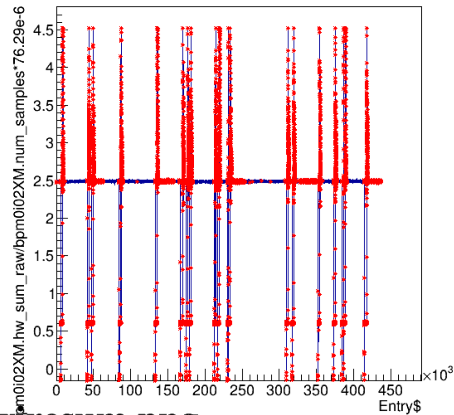
bpm0i02XM.hw_sum_raw/bpm0i02XM.num_samples*76.29e-6:Entry$
