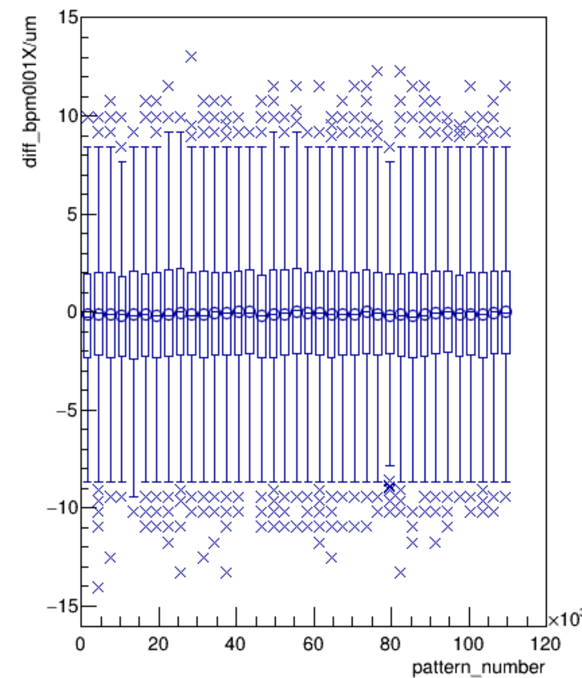
diff_bpm0l01X/um:pattern_number (ErrorFlag==0)
