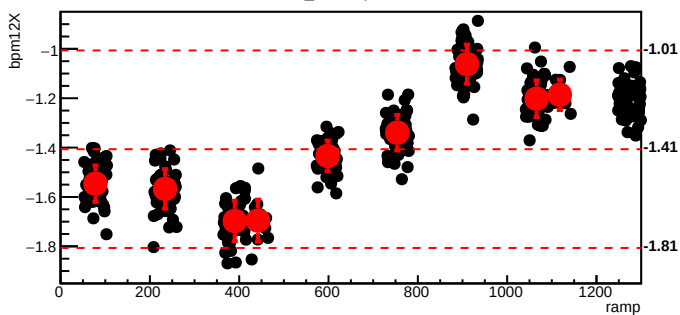
bmod_trim7,cyc=10550
