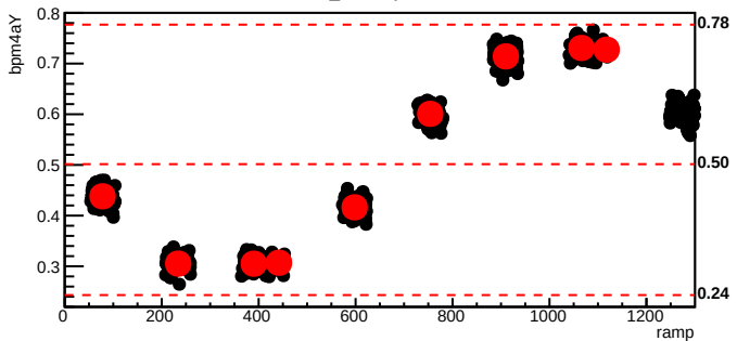
bmod_trim6,cyc=10550
