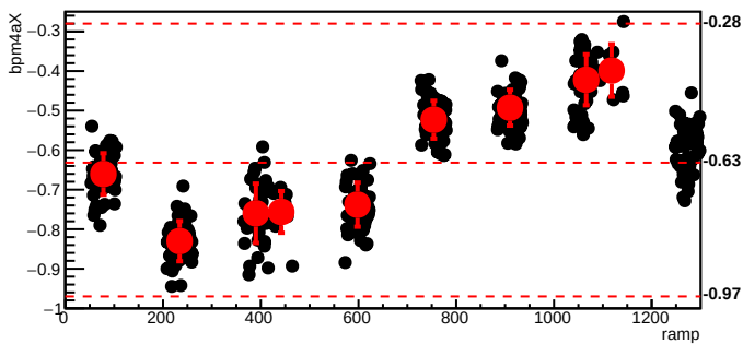
bmod_trim1,cyc=10550
