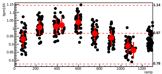
bmod_trim3,cyc=10550
