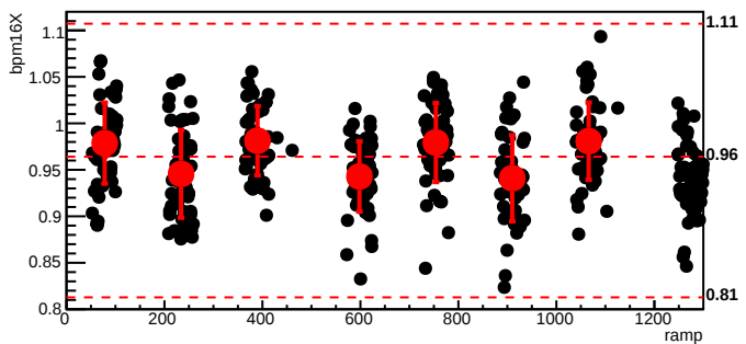
bmod_trim2,cyc=10552
