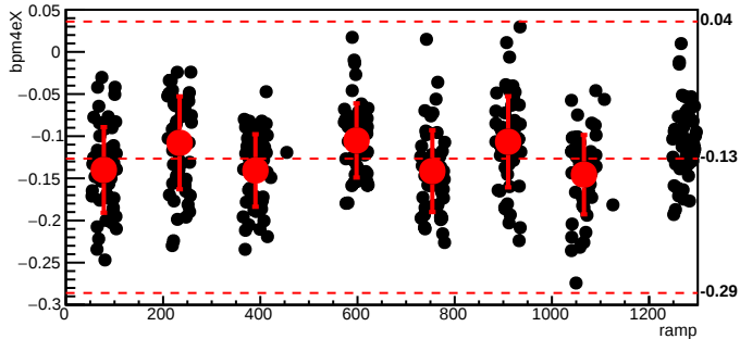
bmod_trim2,cyc=10552
