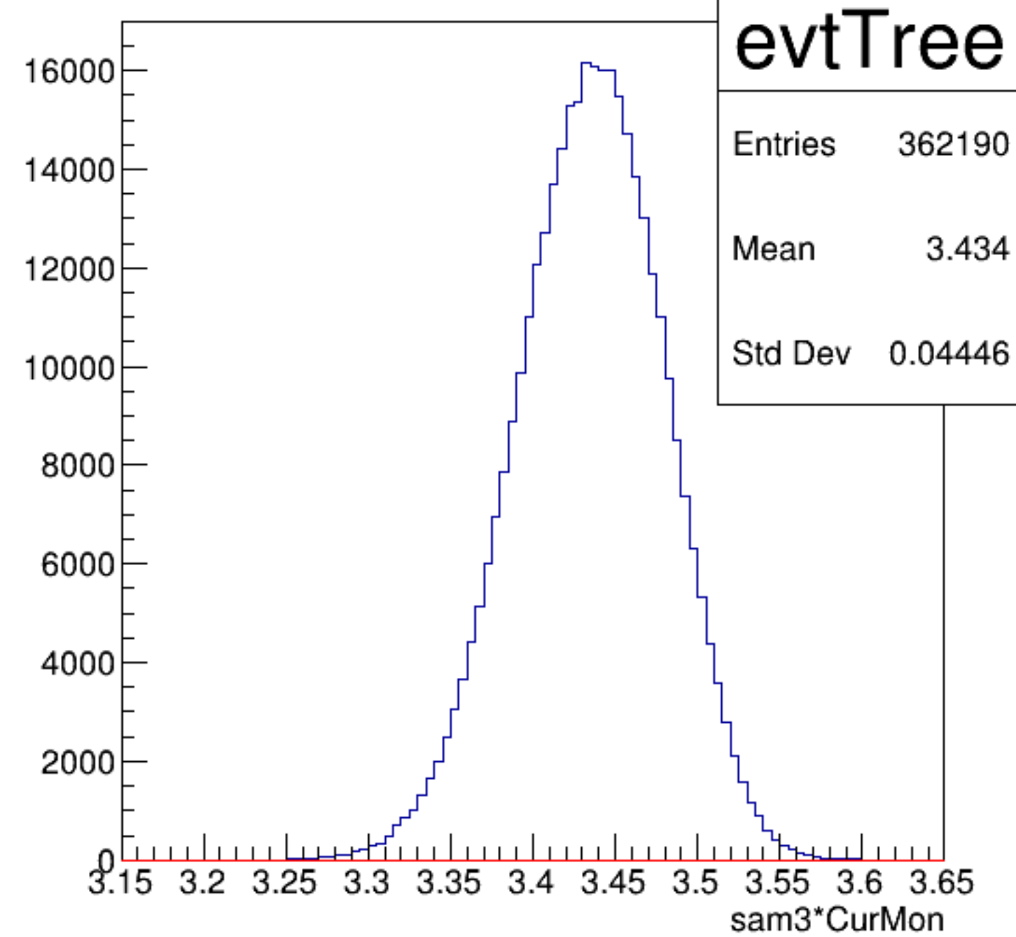
sam3*CurMon {ErrorFlag==0}
