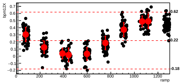
bmod_trim3,cyc=10722
