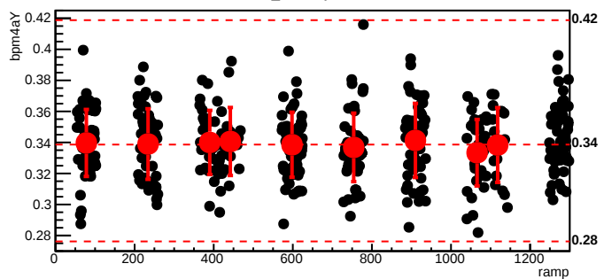
bmod_trim7,cyc=10722
