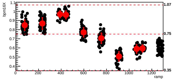
bmod_trim1,cyc=10722
