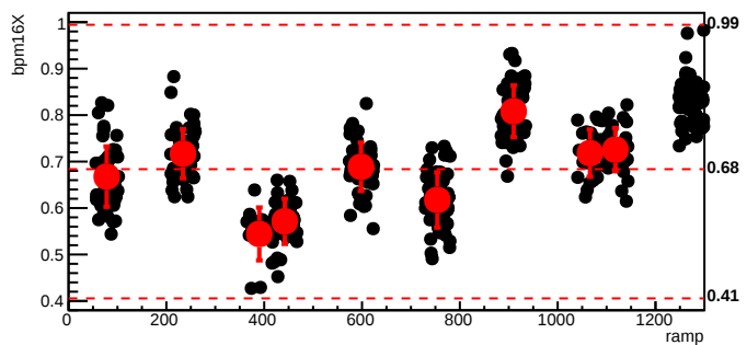
bmod_trim5,cyc=10722
