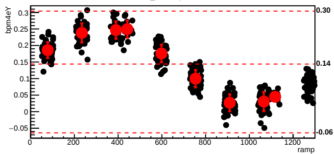
bmod_trim4,cyc=10722
