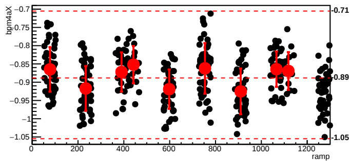
bmod_trim6,cyc=10722
