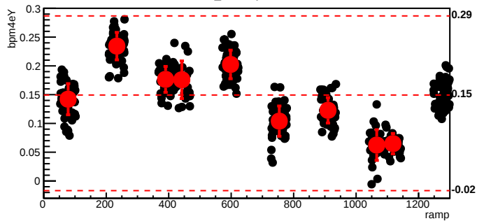
bmod_trim2,cyc=10722
