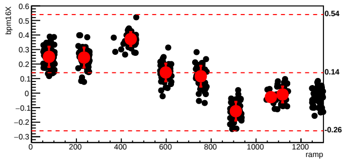
bmod_trim1,cyc=10766
