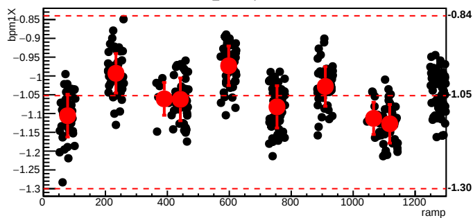
bmod_trim3,cyc=10766
