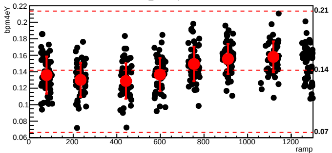
bmod_trim7,cyc=10766
