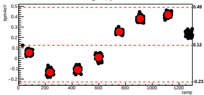
bmod_trim6,cyc=10791
