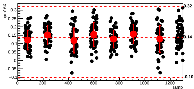
bmod_trim2,cyc=10791
