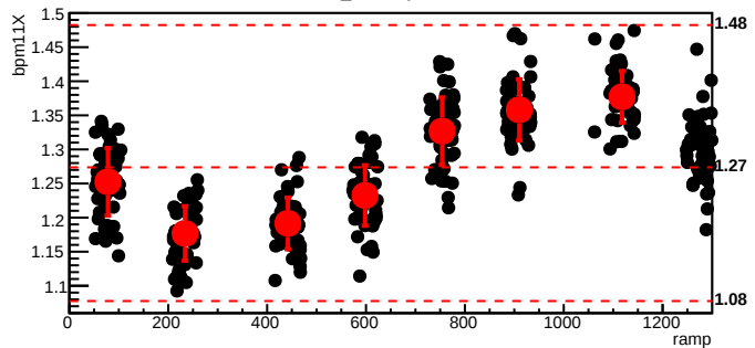
bmod_trim7,cyc=10791
