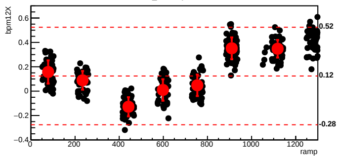
bmod_trim3,cyc=10791
