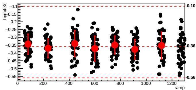
bmod_trim2,cyc=10791
