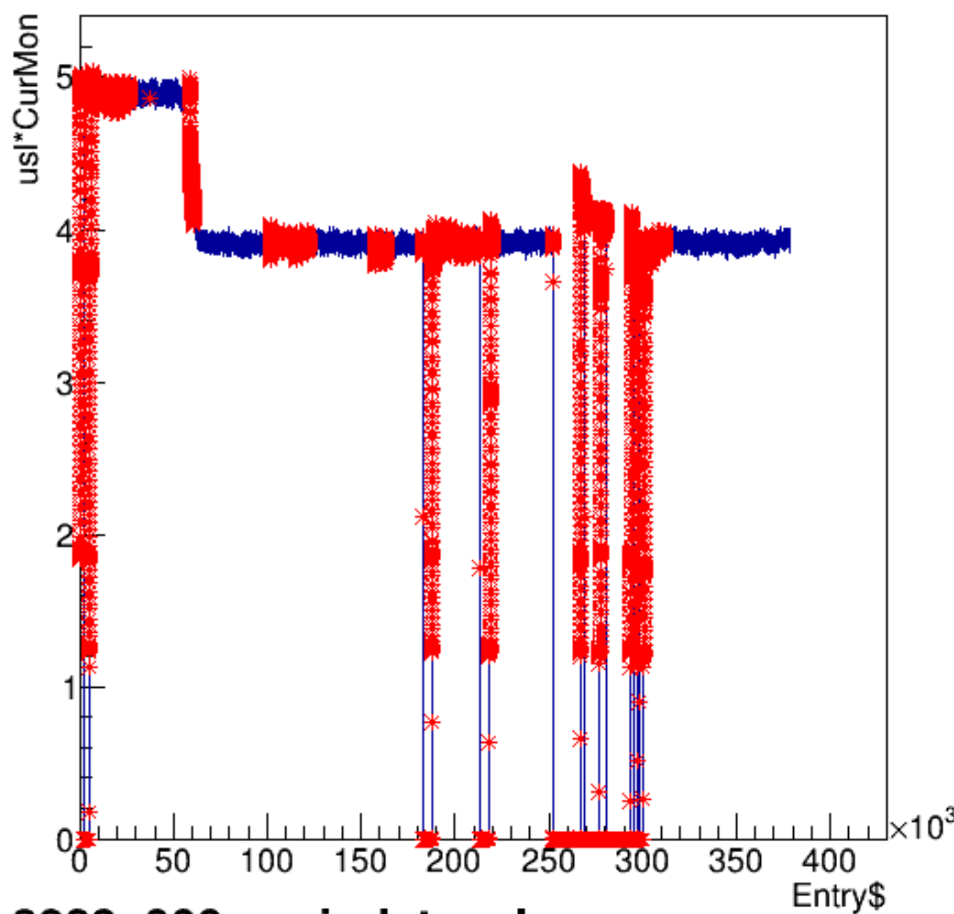
usl*CurMon:Entry$
