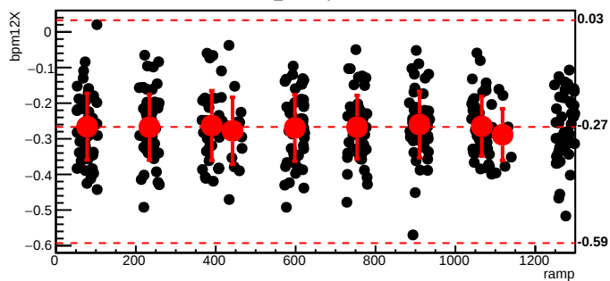
bmod_trim2,cyc=10878
