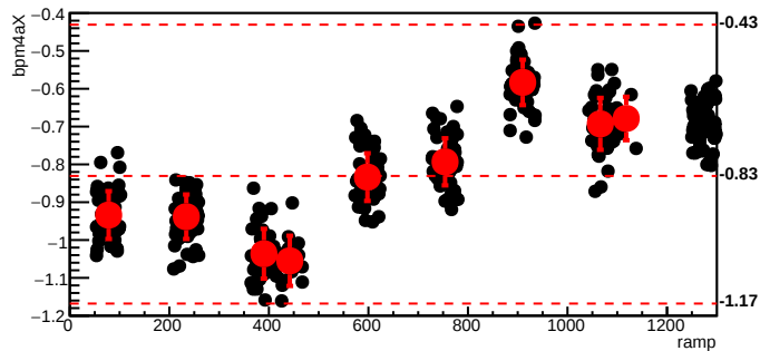
bmod_trim1,cyc=10878
