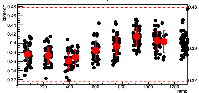
bmod_trim7,cyc=10879
