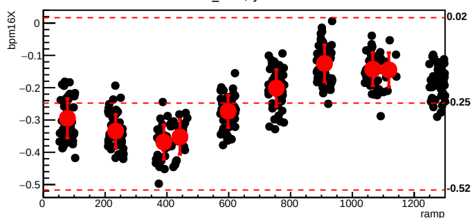
bmod_trim7,cyc=10879
