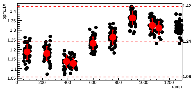
bmod_trim1,cyc=11024
