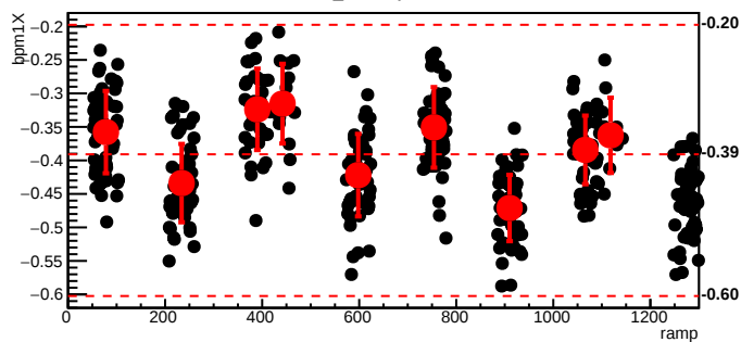
bmod_trim3,cyc=11024
