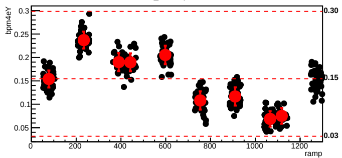
bmod_trim2,cyc=11034
