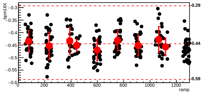
bmod_trim6,cyc=11036
