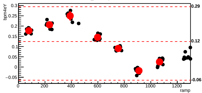
bmod_trim4,cyc=11036
