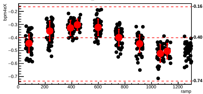
bmod_trim5,cyc=11040
