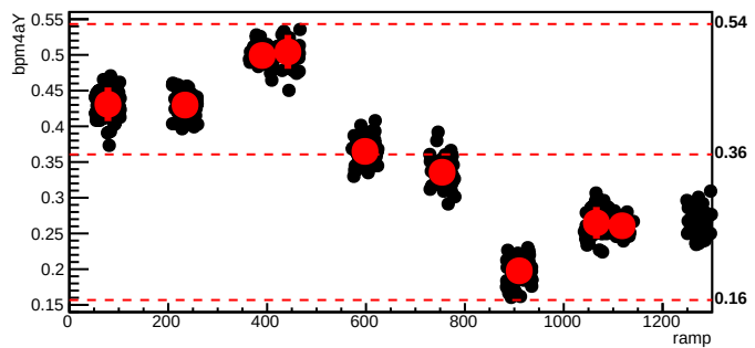
bmod_trim4,cyc=11040
