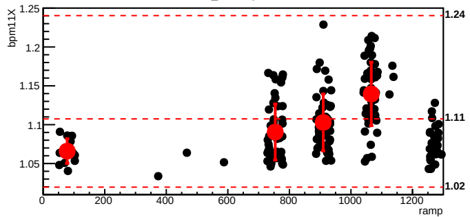
bmod_trim7,cyc=11040
