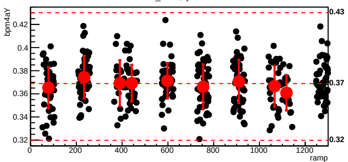
bmod_trim1,cyc=11040
