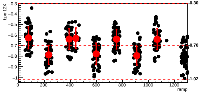
bmod_trim4,cyc=11041
