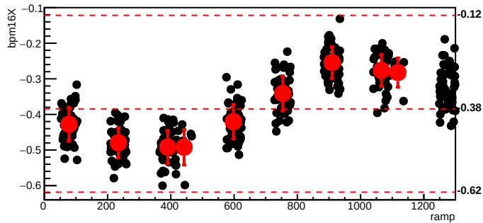
bmod_trim7,cyc=11041
