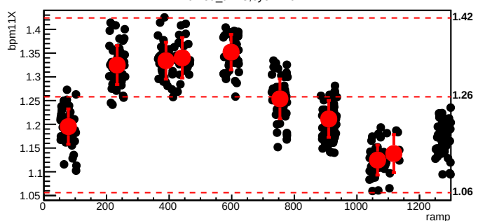
bmod_trim5,cyc=11041
