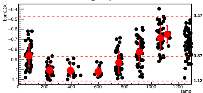
bmod_trim3,cyc=11041
