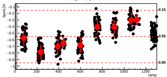
bmod_trim1,cyc=11041
