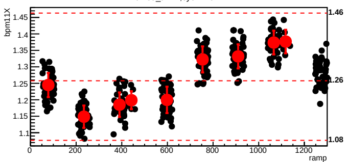
bmod_trim1,cyc=11041
