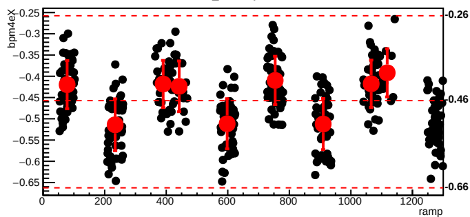
bmod_trim6,cyc=11041
