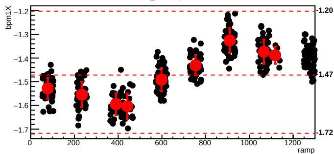
bmod_trim1,cyc=11076
