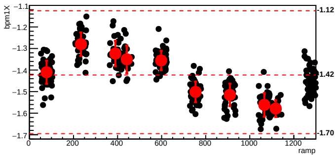
bmod_trim7,cyc=11076
