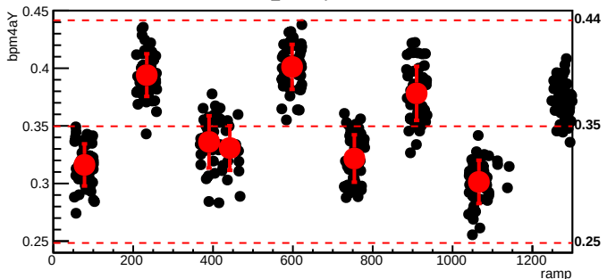
bmod_trim3,cyc=11076
