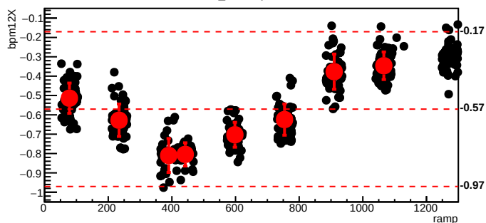
bmod_trim3,cyc=11076
