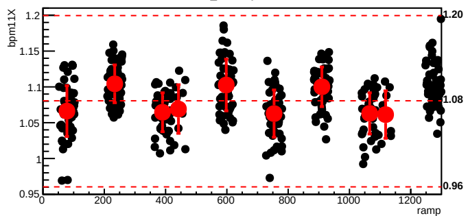
bmod_trim2,cyc=11076
