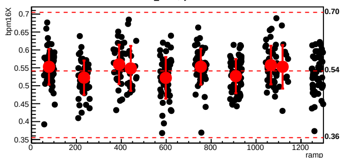
bmod_trim4,cyc=11076
