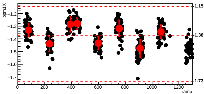
bmod_trim3,cyc=11076
