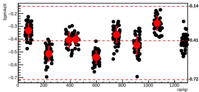
bmod_trim3,cyc=11076
