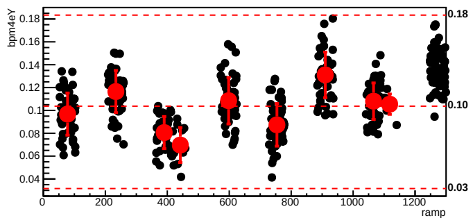
bmod_trim5,cyc=11076
