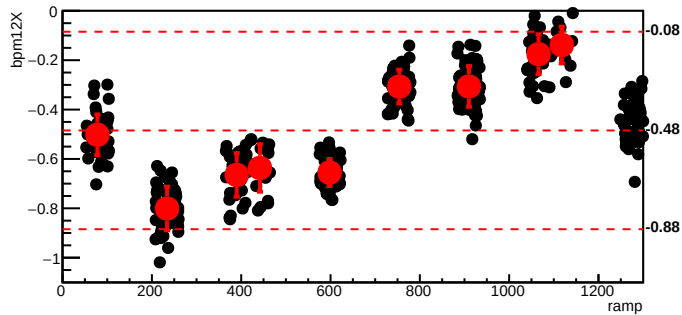
bmod_trim7,cyc=11076
