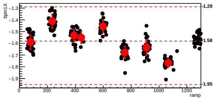
bmod_trim7,cyc=11077
