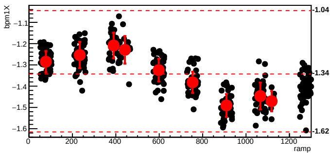
bmod_trim7,cyc=11080
