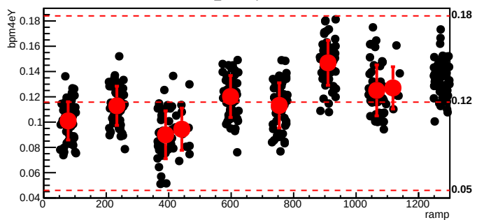
bmod_trim7,cyc=11080
