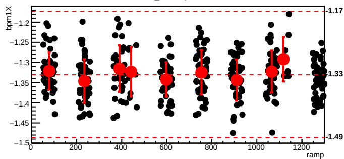
bmod_trim6,cyc=11080
