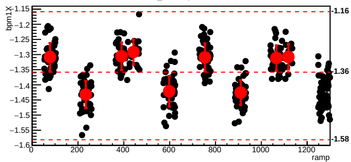
bmod_trim6,cyc=11087
