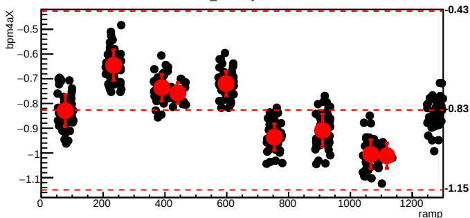
bmod_trim7,cyc=11087
