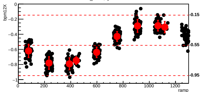
bmod_trim7,cyc=11087
