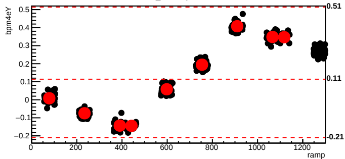
bmod_trim6,cyc=11101
