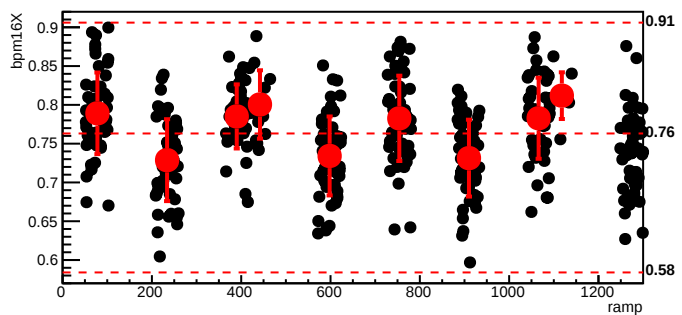
bmod_trim4,cyc=11101
