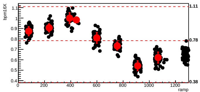
bmod_trim1,cyc=11101
