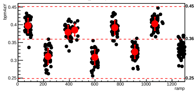
bmod_trim5,cyc=11104
