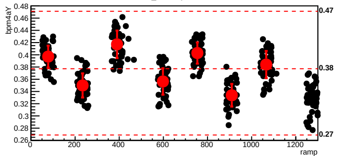
bmod_trim3,cyc=11104
