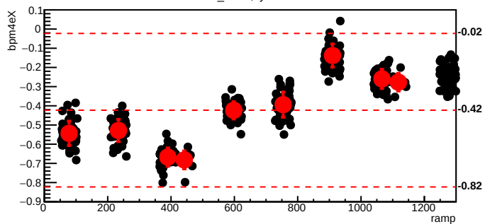
bmod_trim1,cyc=11104
