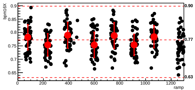
bmod_trim4,cyc=11104
