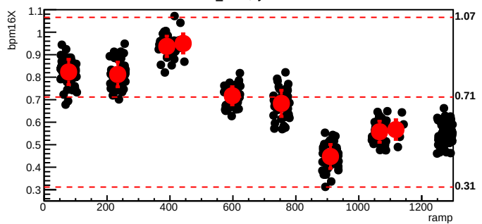
bmod_trim1,cyc=11104
