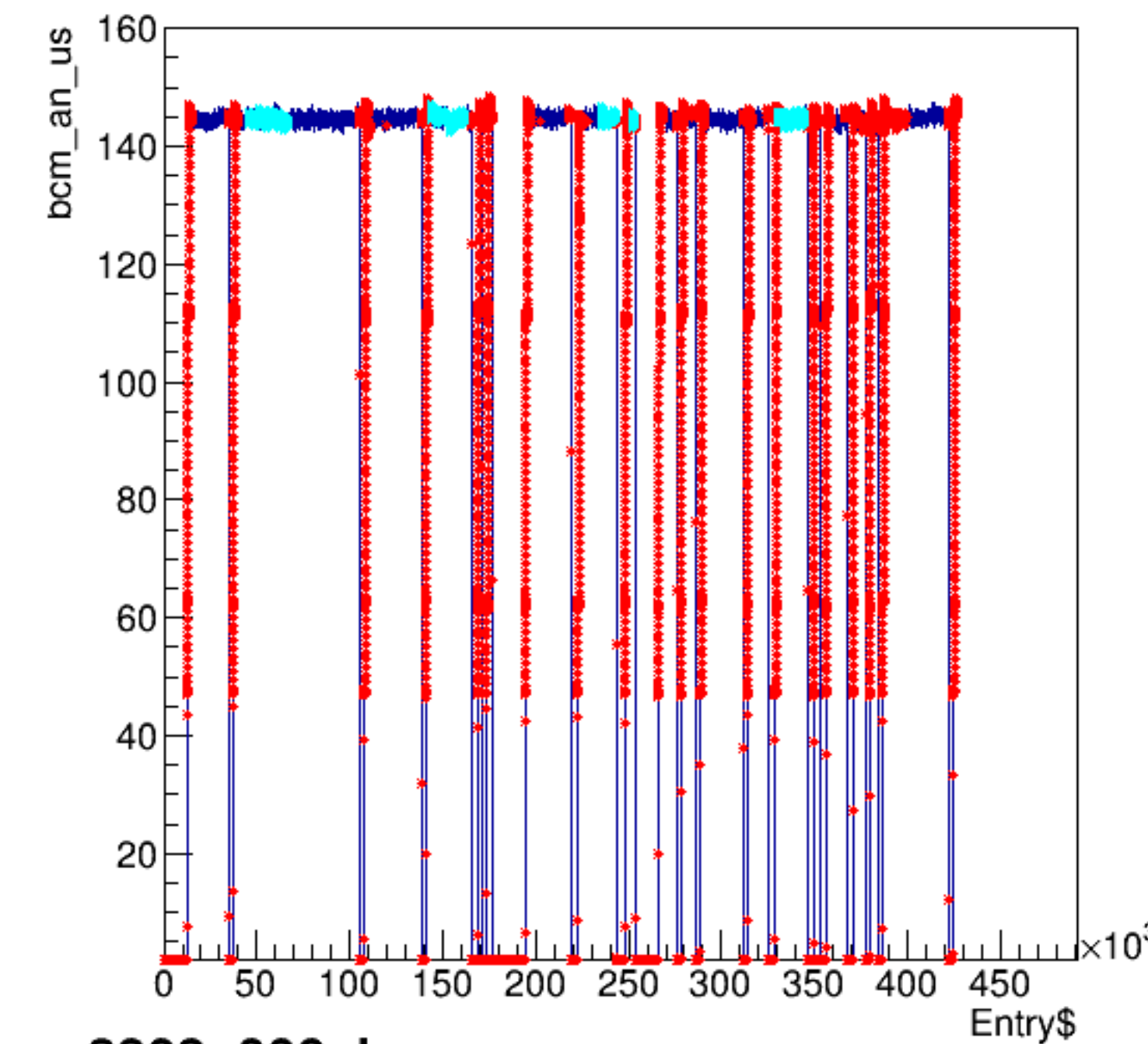
bcm_an_us:Entry$
