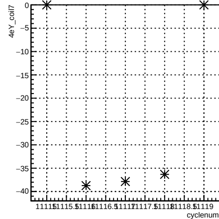
4eY_coil7:cyclenum {run == 8305}
