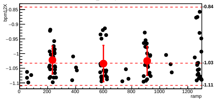
bmod_trim2,cyc=11115
