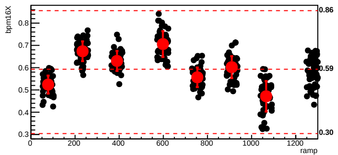
bmod_trim3,cyc=11115
