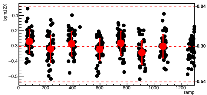
bmod_trim6,cyc=11115
