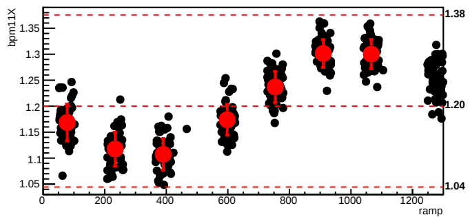
bmod_trim1,cyc=11115
