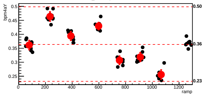
bmod_trim2,cyc=11119
