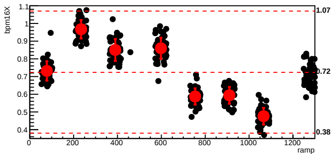
bmod_trim1,cyc=11119
