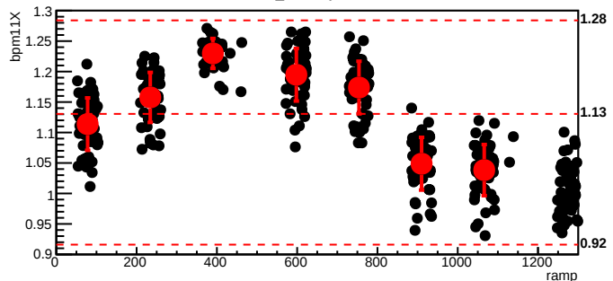
bmod_trim5,cyc=11147
