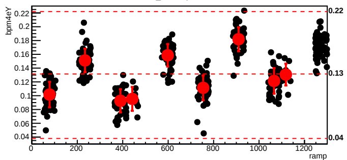
bmod_trim7,cyc=11147
