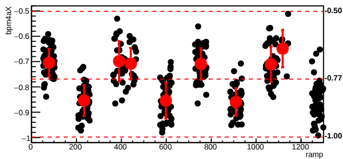
bmod_trim6,cyc=11147
