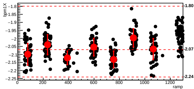
bmod_trim5,cyc=11147
