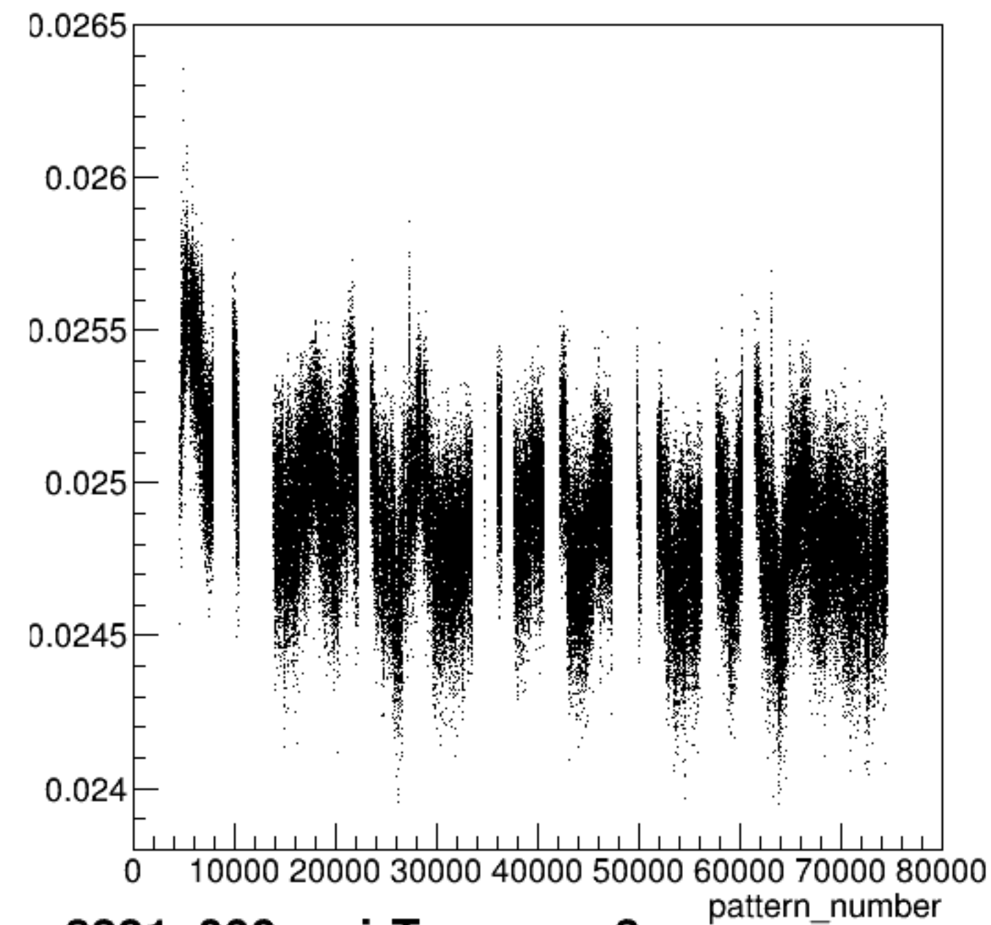
yield_sam3:pattern_number {ErrorFlag==0}
