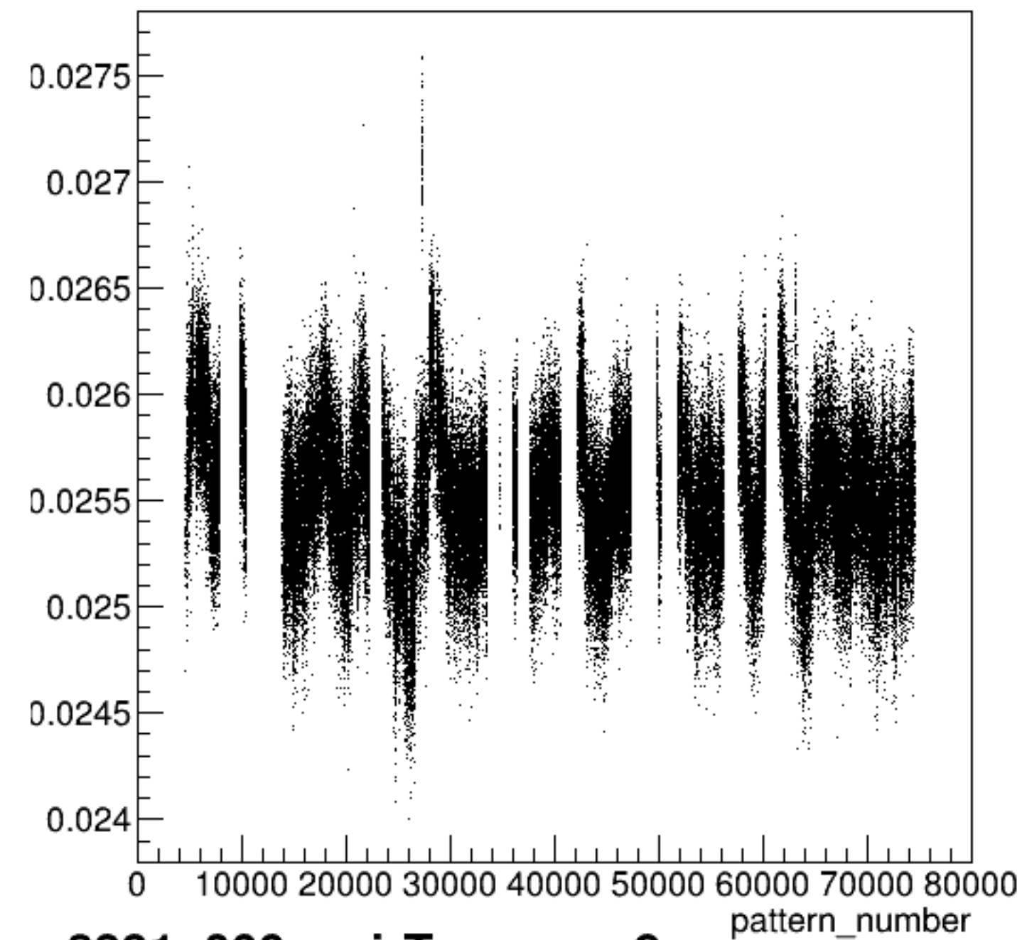
yield_sam2:pattern_number {ErrorFlag==0}
