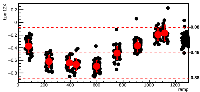
bmod_trim3,cyc=11249
