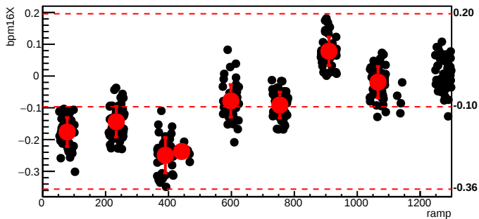
bmod_trim7,cyc=11251
