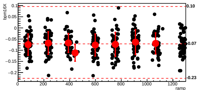
bmod_trim2,cyc=11251
