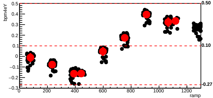
bmod_trim6,cyc=11251
