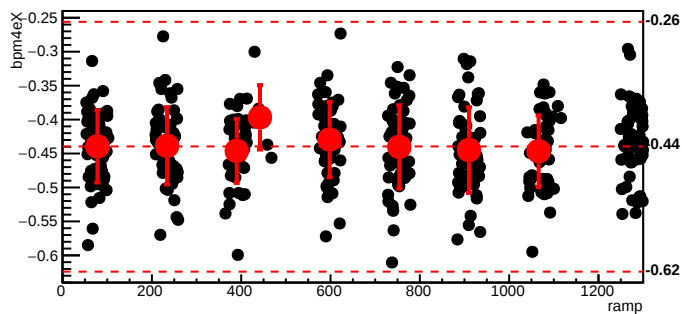
bmod_trim2,cyc=11251
