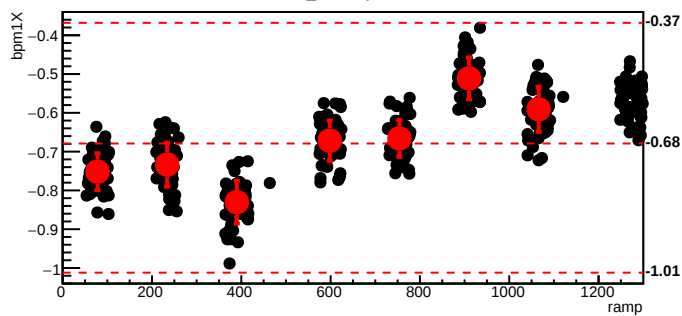
bmod_trim1,cyc=11364
