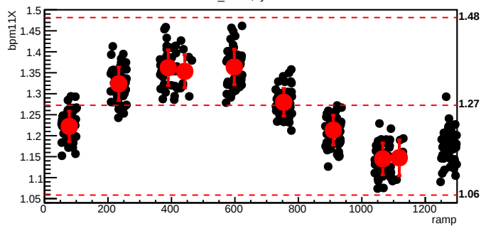
bmod_trim5,cyc=11364
