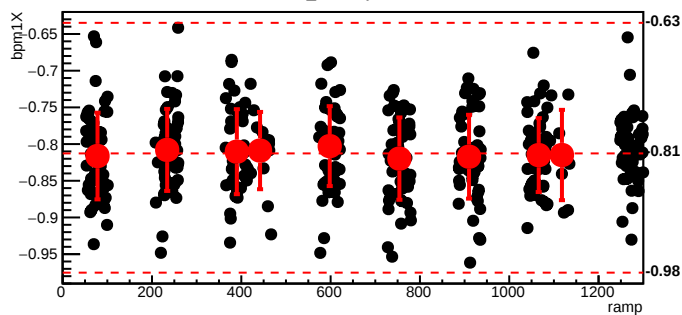
bmod_trim6,cyc=11364
