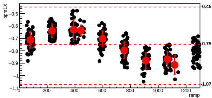
bmod_trim7,cyc=11364
