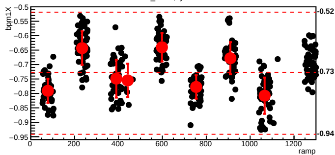
bmod_trim3,cyc=11365
