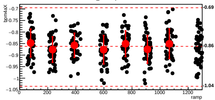
bmod_trim6,cyc=11365
