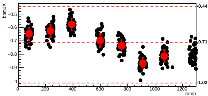
bmod_trim7,cyc=11365
