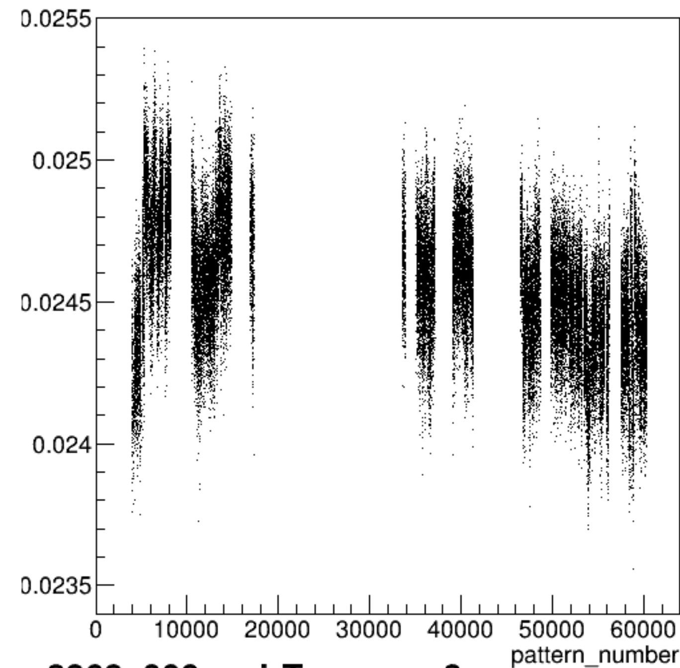
yield_sam3:pattern_number {ErrorFlag==0}
