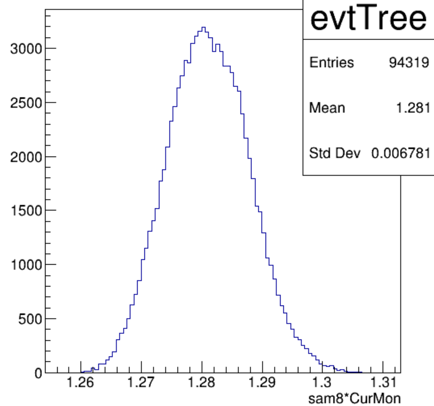
sam8*CurMon {ErrorFlag==0}
