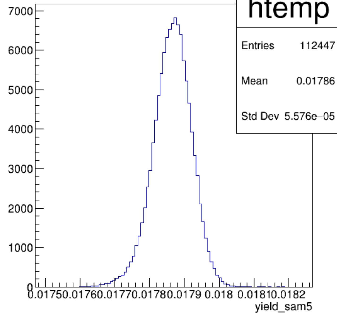
yield_sam5 {ErrorFlag==0}
