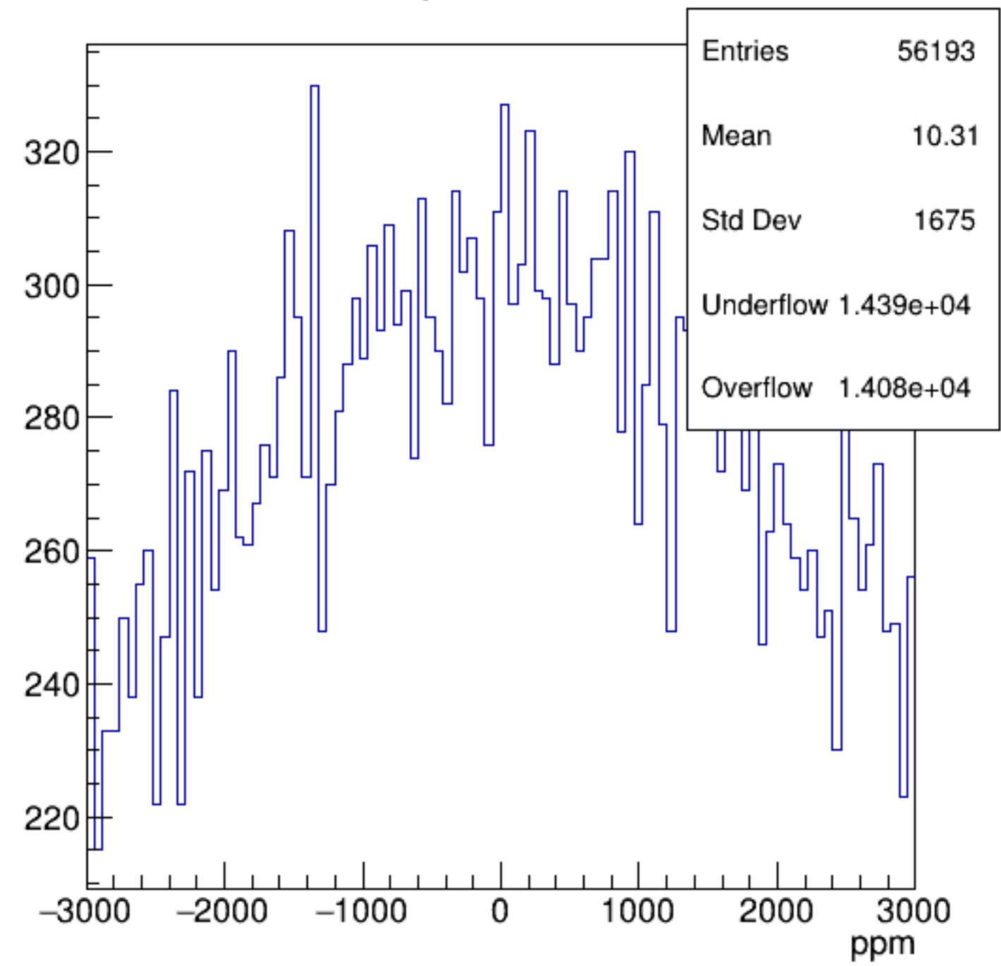
asym_sam2
