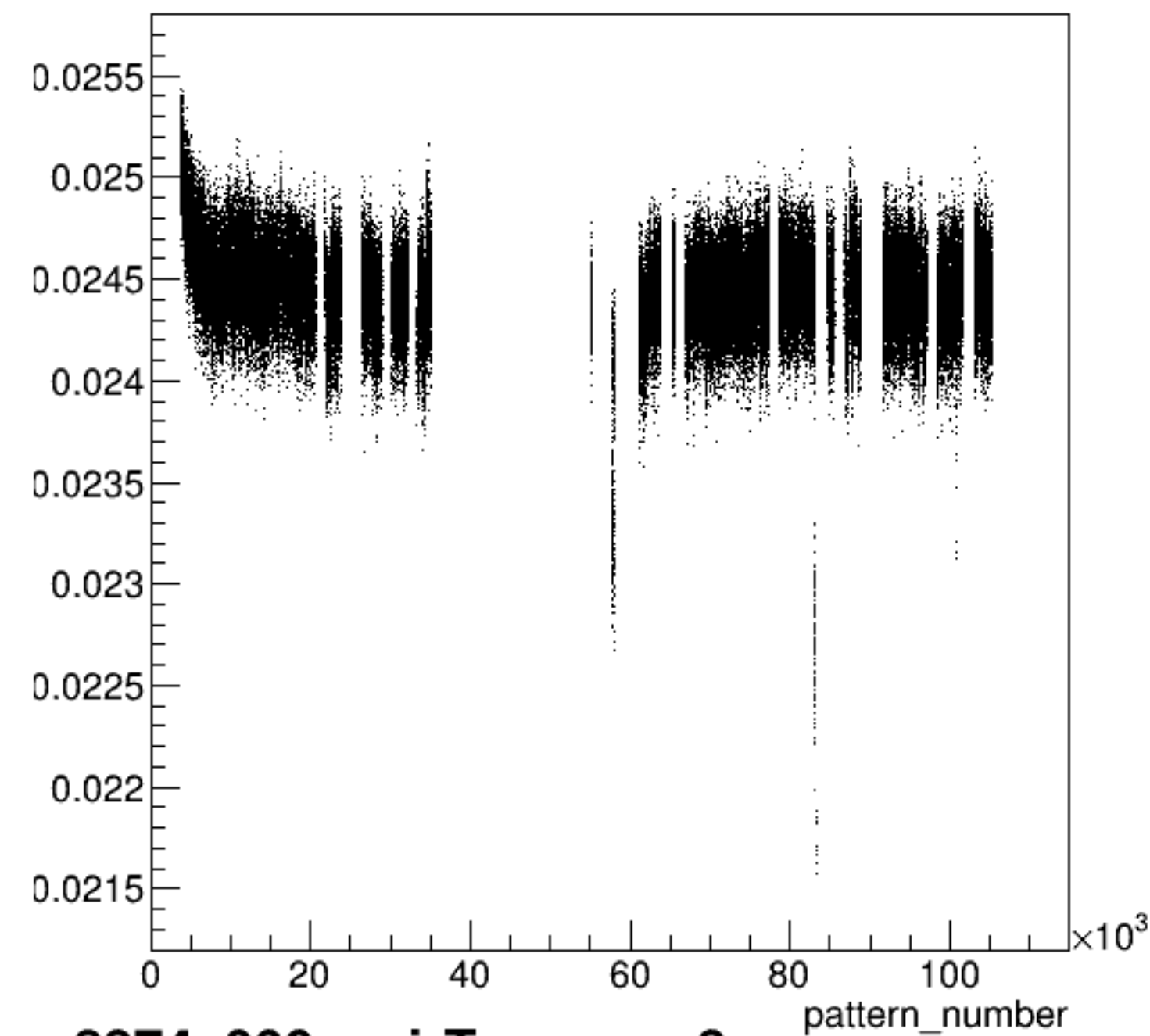
yield_sam3:pattern_number {ErrorFlag==0}
