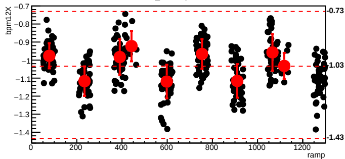
bmod_trim2,cyc=11412
