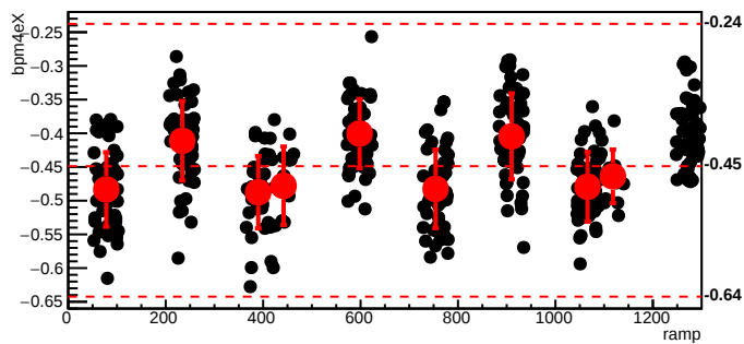
bmod_trim6,cyc=11412
