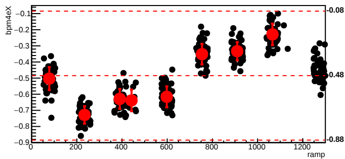
bmod_trim1,cyc=11412
