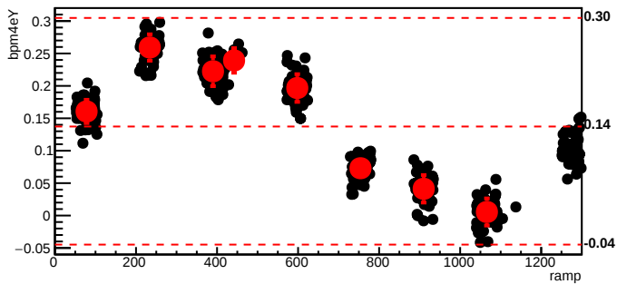
bmod_trim4,cyc=11412
