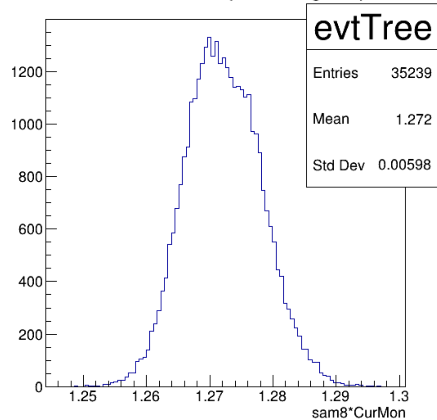
sam8*CurMon {ErrorFlag==0}
