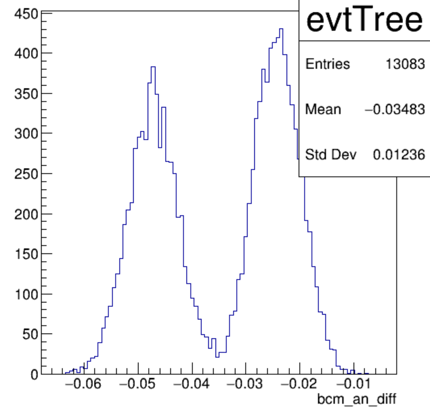
bcm_an_diff {ErrorFlag==0}
