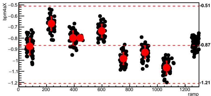
bmod_trim7,cyc=11320
