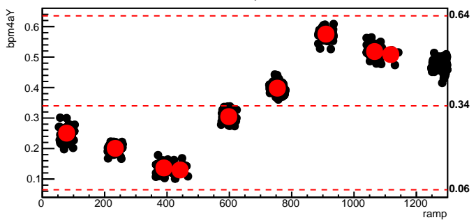
bmod_trim6,cyc=11320
