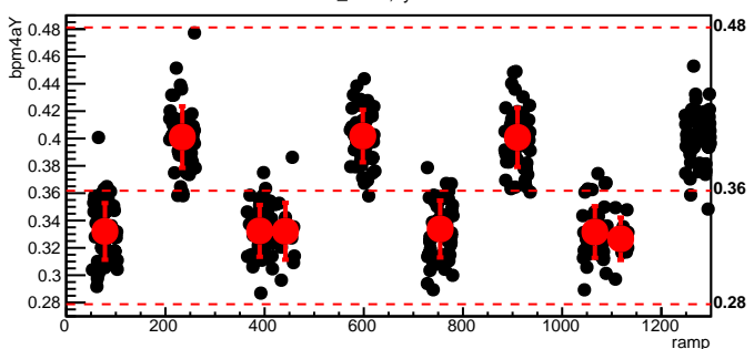
bmod_trim5,cyc=11320
