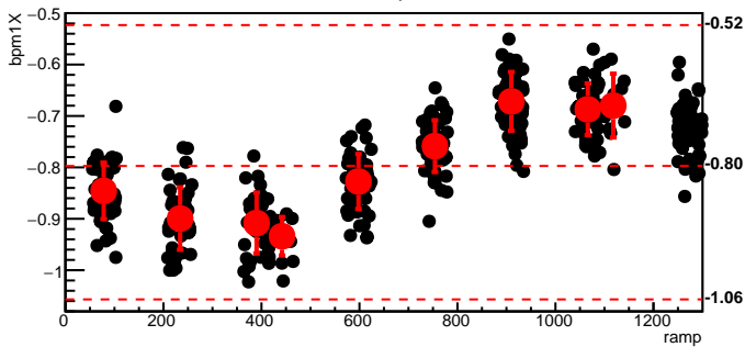
bmod_trim1,cyc=11320
