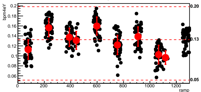
bmod_trim3,cyc=11320
