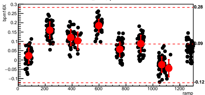
bmod_trim3,cyc=11320
