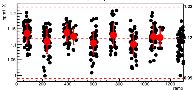
bmod_trim2,cyc=11320
