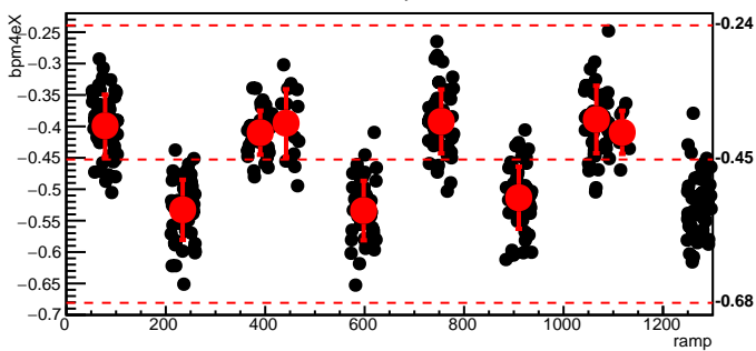
bmod_trim6,cyc=11320
