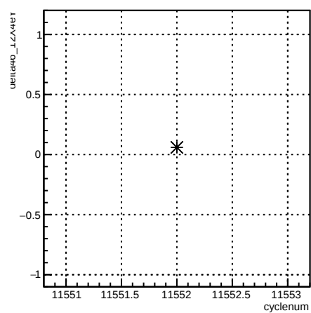
delta46_12X4eY:cyclenum {run == 8407}
