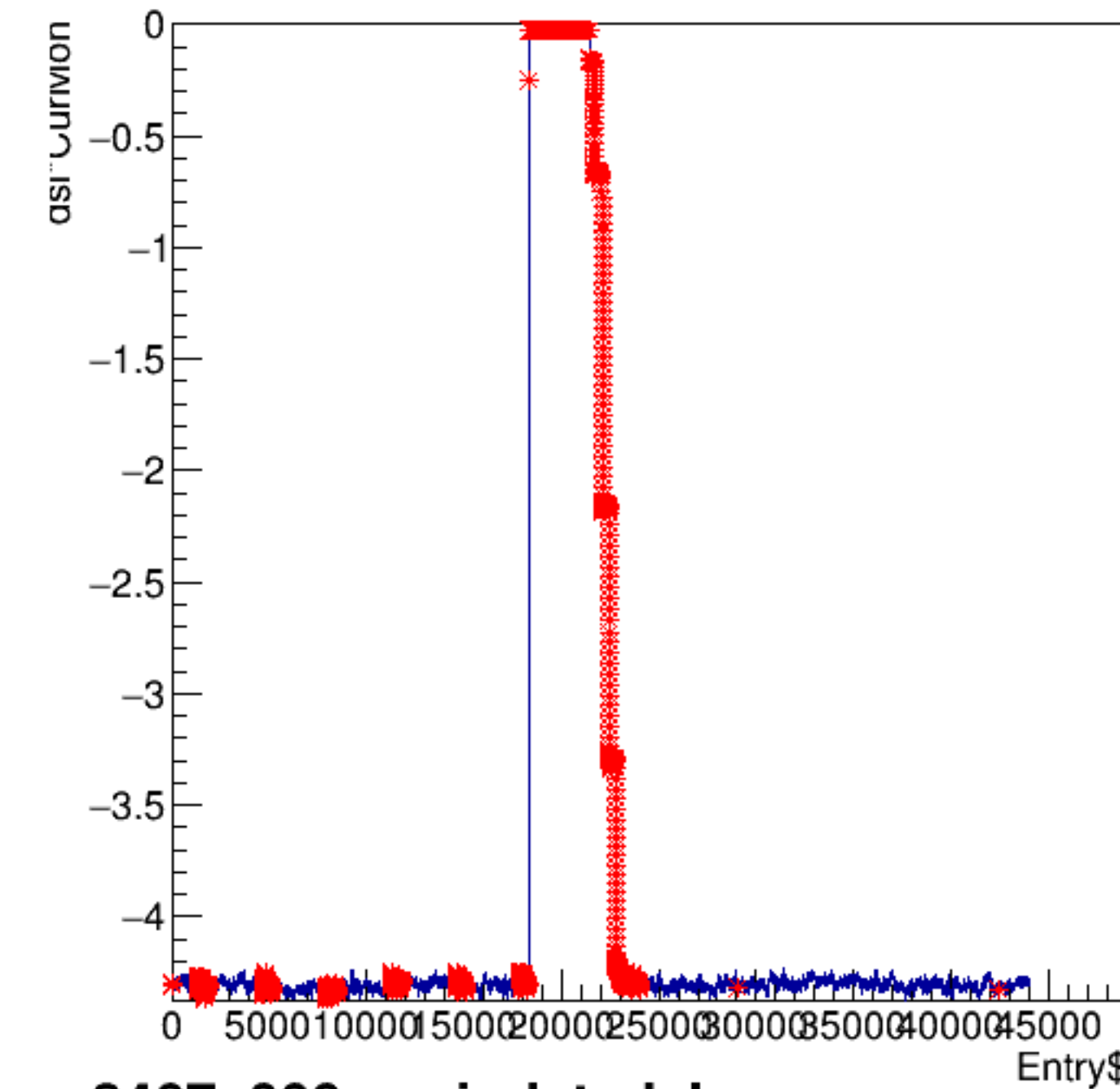
dsl*CurMon:Entry$
