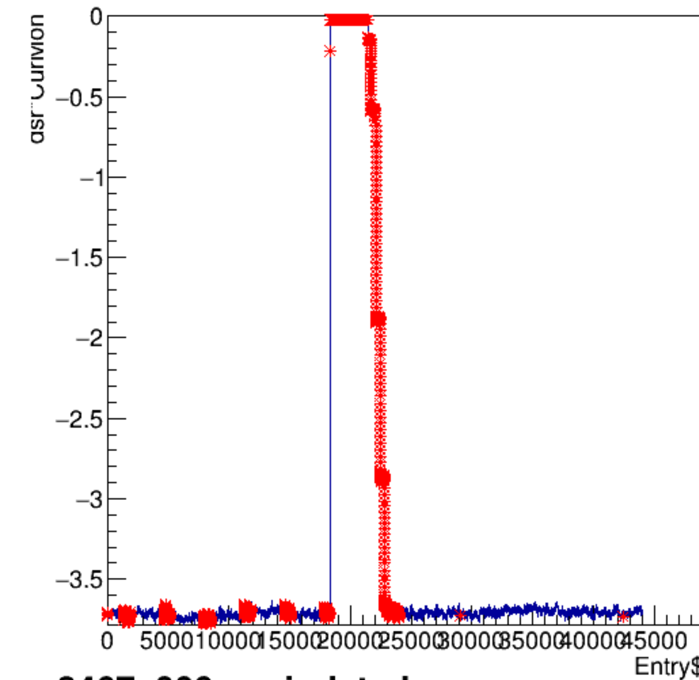
dsr*CurMon:Entry$
