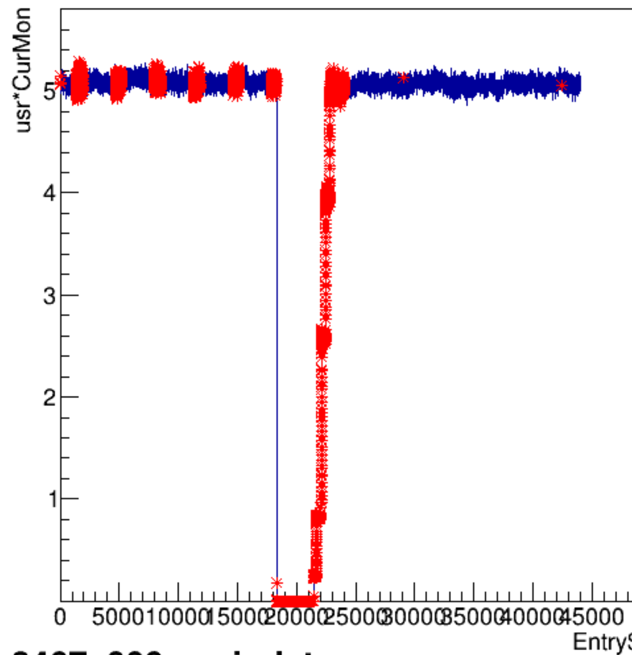
usr*CurMon:Entry$
