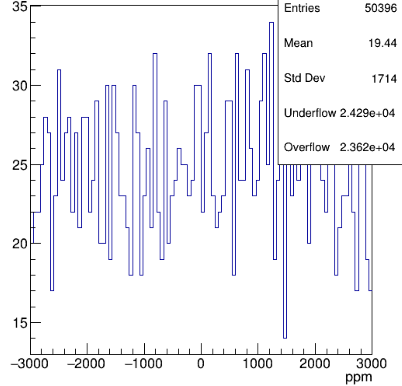
asym_atl2
