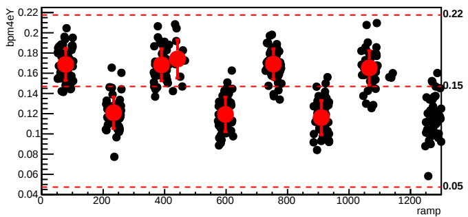
bmod_trim1,cyc=11921
