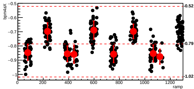
bmod_trim4,cyc=11921
