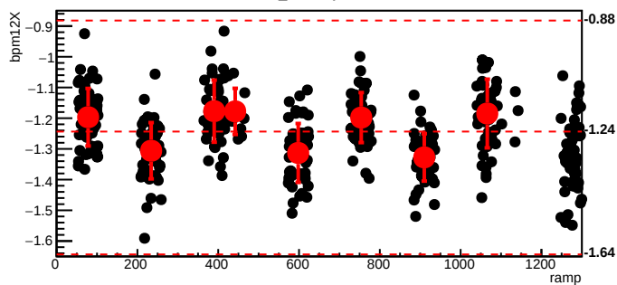
bmod_trim2,cyc=11921
