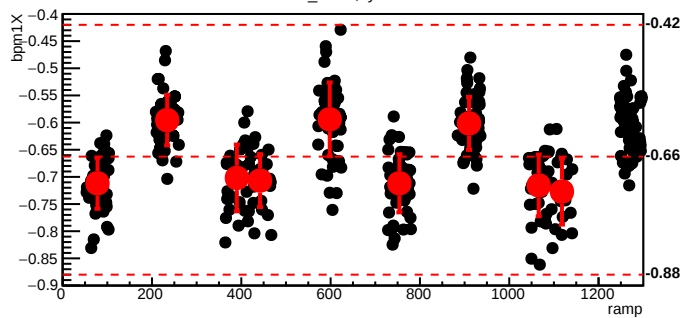
bmod_trim6,cyc=11921
