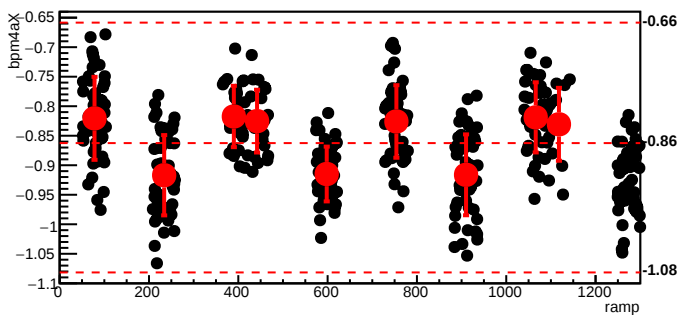
bmod_trim5,cyc=11921
