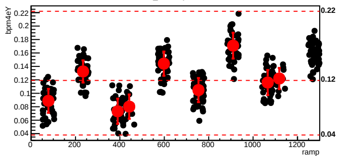
bmod_trim7,cyc=11921
