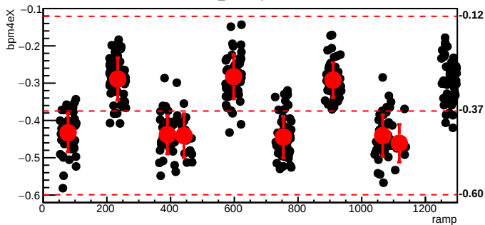
bmod_trim4,cyc=11921
