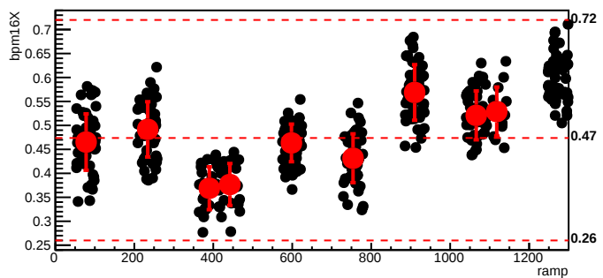
bmod_trim5,cyc=11921
