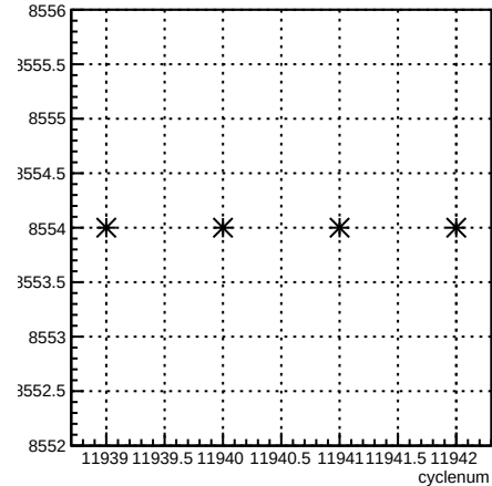
run:cyclenum {run == 8554}
