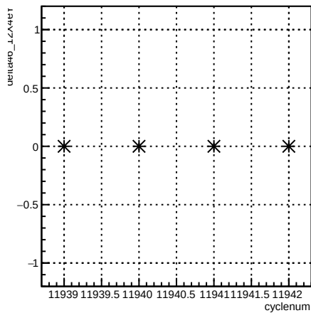
delta46_12X4eY:cyclenum {run == 8554}
