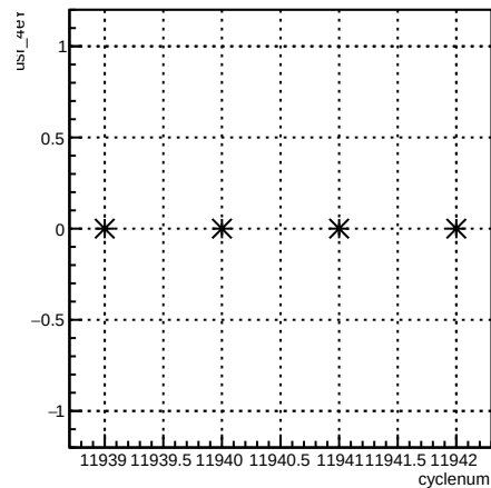
usr_4eY:cyclenum {run == 8554}
