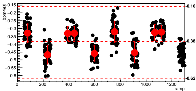
bmod_trim6,cyc=11960
