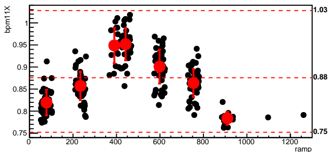
bmod_trim5,cyc=11960
