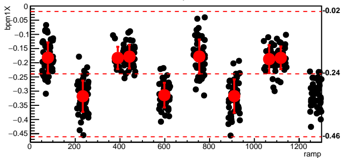
bmod_trim6,cyc=11960
