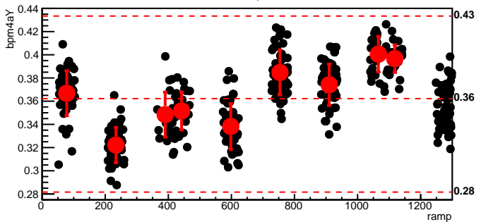
bmod_trim7,cyc=11960
