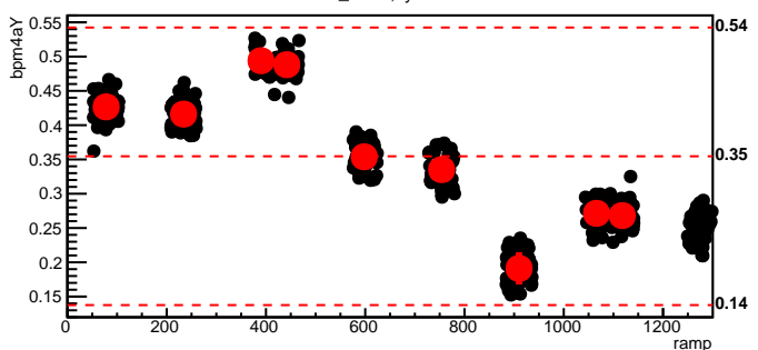
bmod_trim4,cyc=11960
