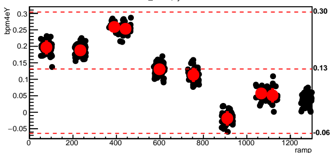
bmod_trim4,cyc=11960
