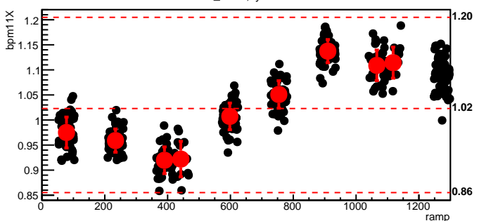
bmod_trim1,cyc=11960
