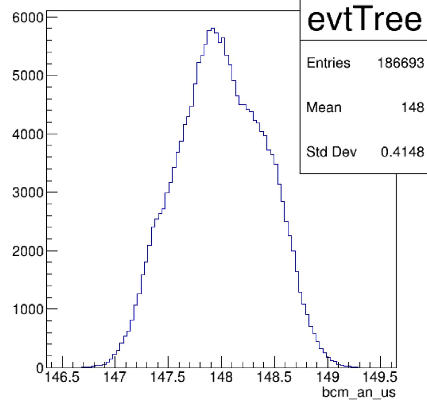
bcm_an_us {ErrorFlag==0}
