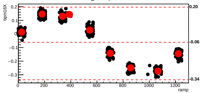
bmod_trim1,cyc=6014
