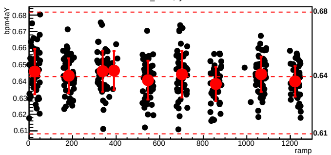
bmod_trim1,cyc=6014
